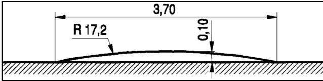
3.2. Próg płytowy z powierzchniami najazdowymi łukowymi (U-16b)
