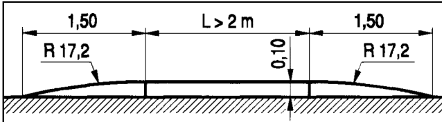
3.3. Próg płytowy z powierzchniami najazdowymi ukośnymi (U-16c)
