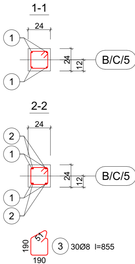
Wykaz zbrojenia
