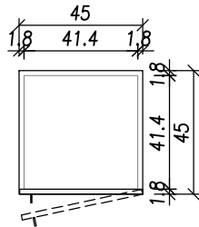
PRZEKRÓJ B-B
