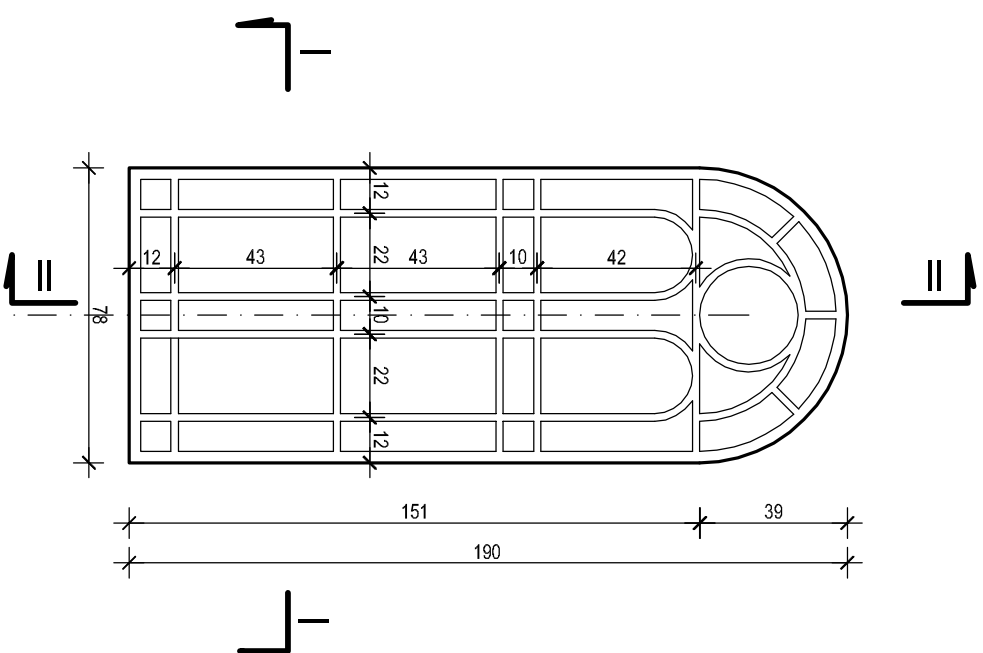
widok okna od zewnątrz 1:20
