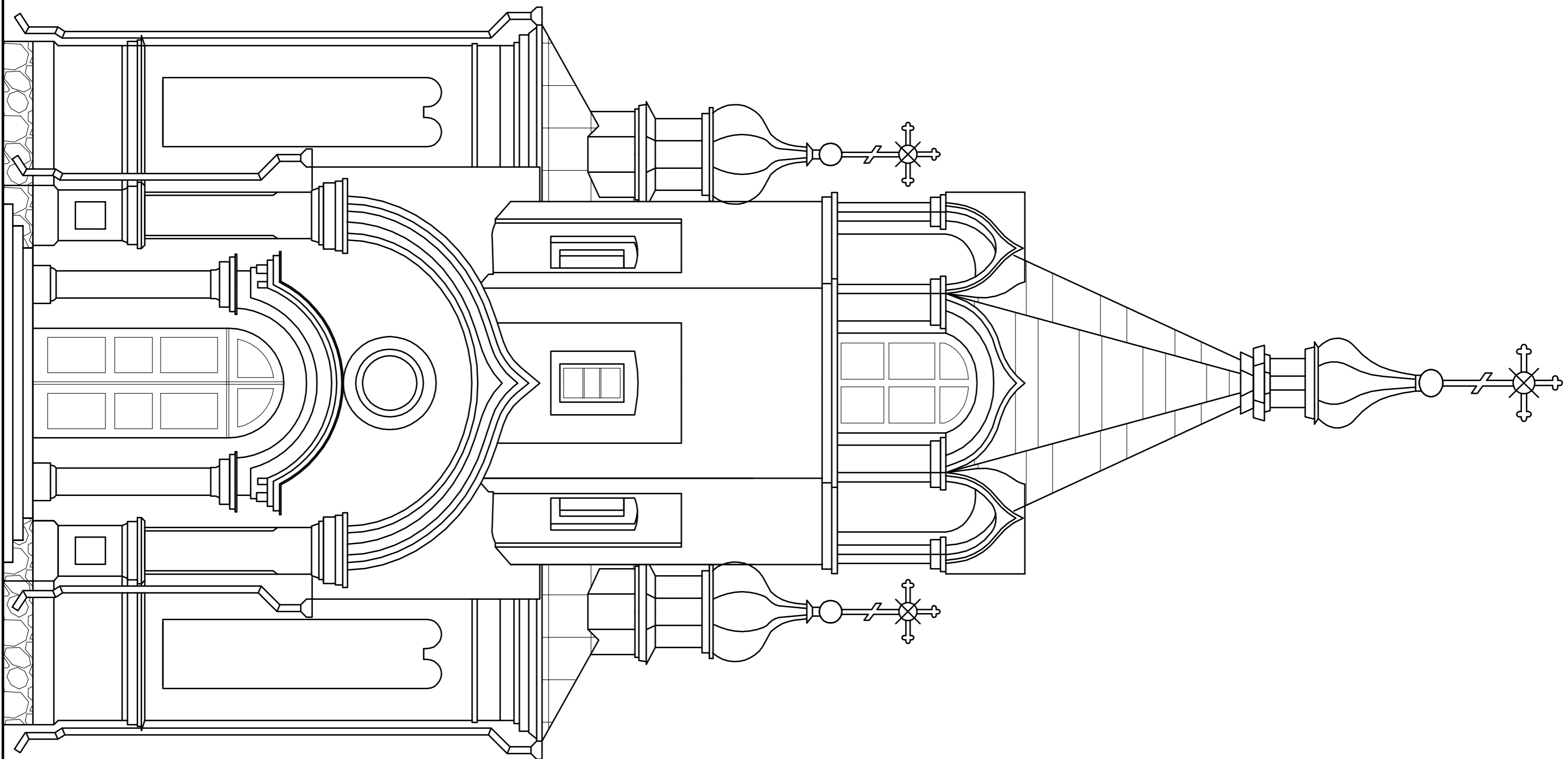
ELEWACJA PÓŁNOCNO-ZACHODNIA
