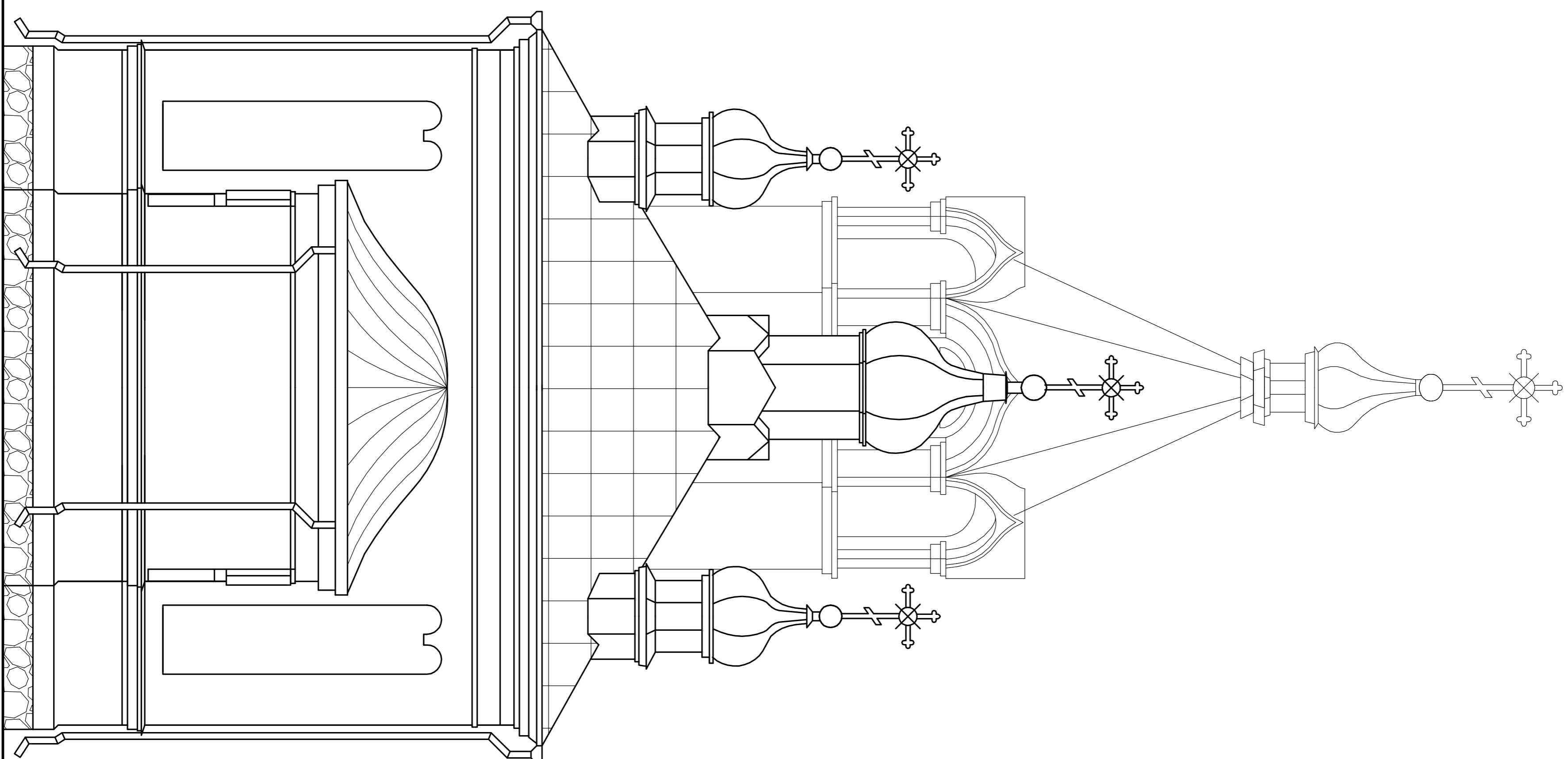
ELEWACJA PÓŁDNIOWO-WSCHODNIA
