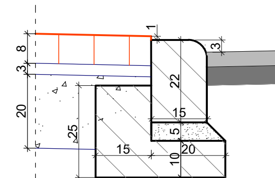
Krawężnik betonowy najazdowy 22x15x100 na ławie betonowej z oporem z betonu C12/15
