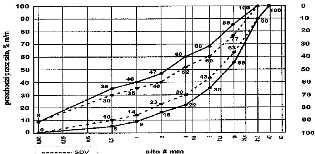
Rys. 2.1 Krzywe graniczne uziarnienia mieszanki niezwiązanej 0/31,5 mm do warstw podbudowy zasadniczej
