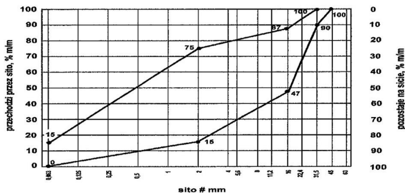
Rys. 1 Mieszanka niezwiązana 0/31,5 do nawierzchni z kruszywa niezwiązanego
