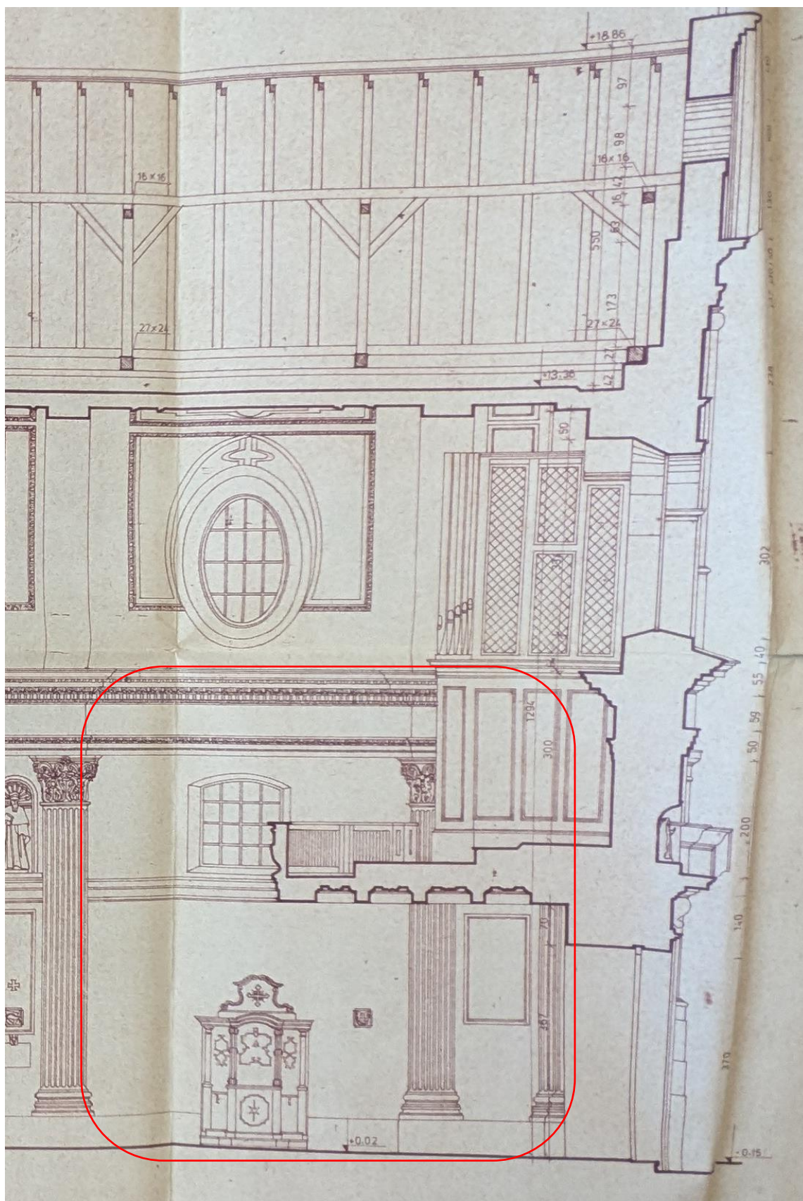
Rys. nr 3 – Przekrój pionowy budynku nr 1 – część przewidziana do czyszczenia
