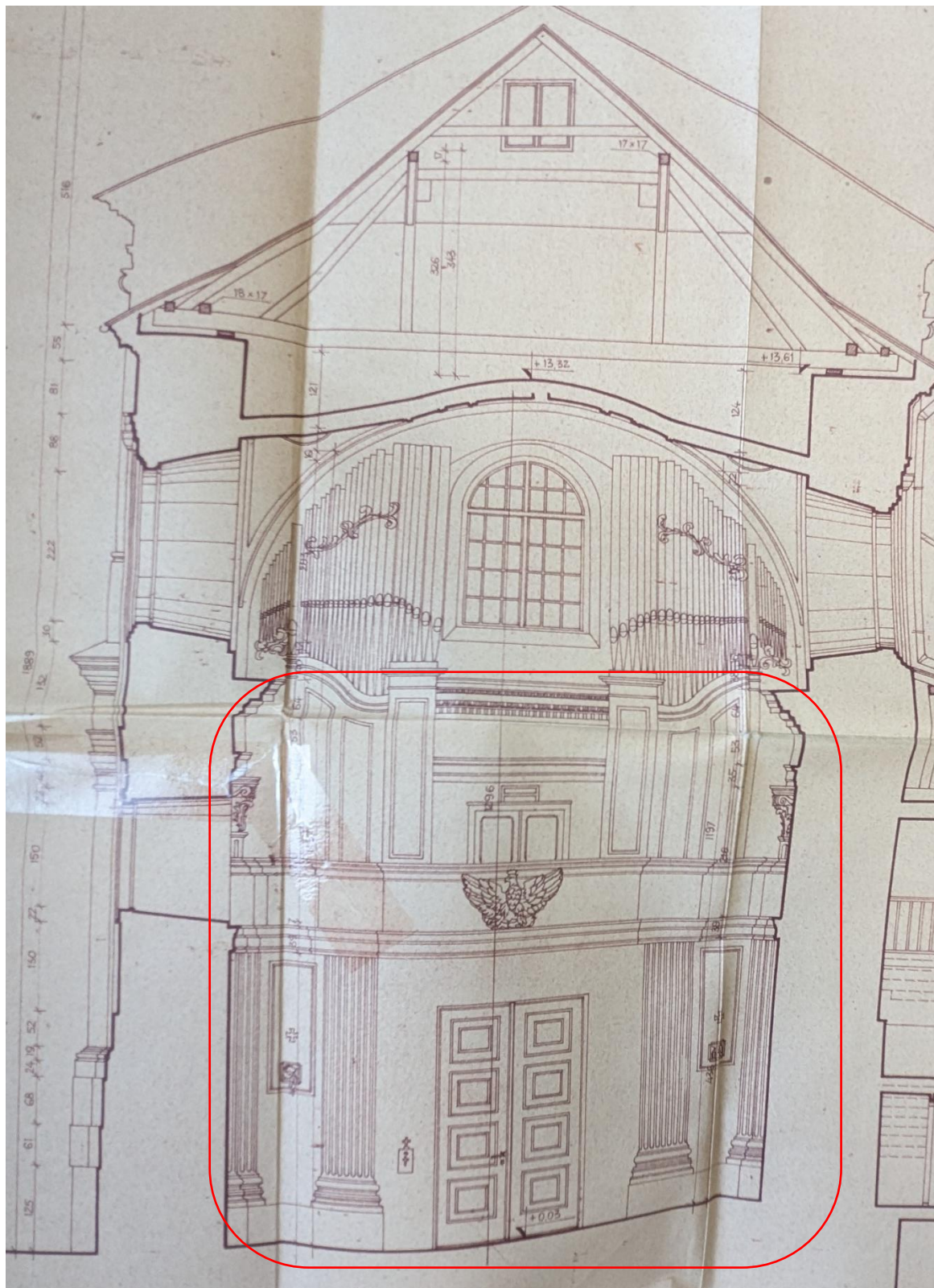
Rys. nr 4 – Przekrój pionowy budynku nr 1 – część przewidziana do czyszczenia
