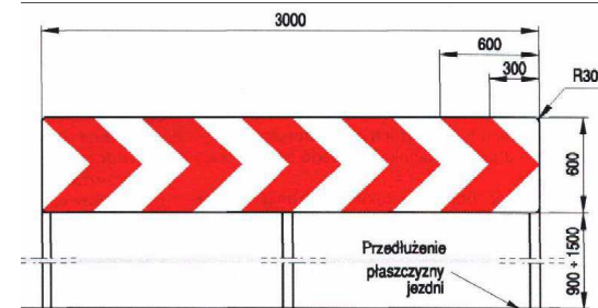
Rys. 4. Zapora drogowa podwójna
