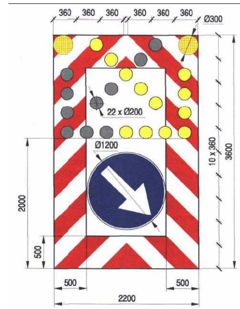
Rys. 15. Wzór tablicy zamykającej U-26a
