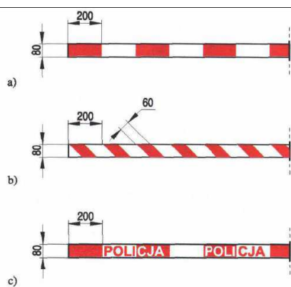
Rys. 8. Przykłady taśm ostrzegawczych U-22
