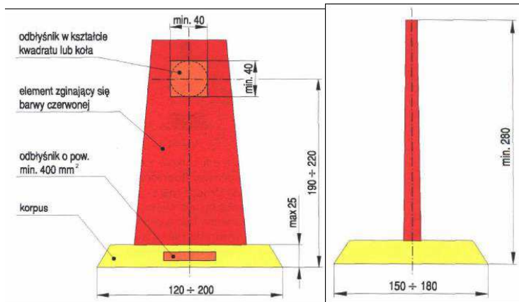
Rys. 12. Przykład separatora ruchu ciągłego U-25a barwy żółtej
