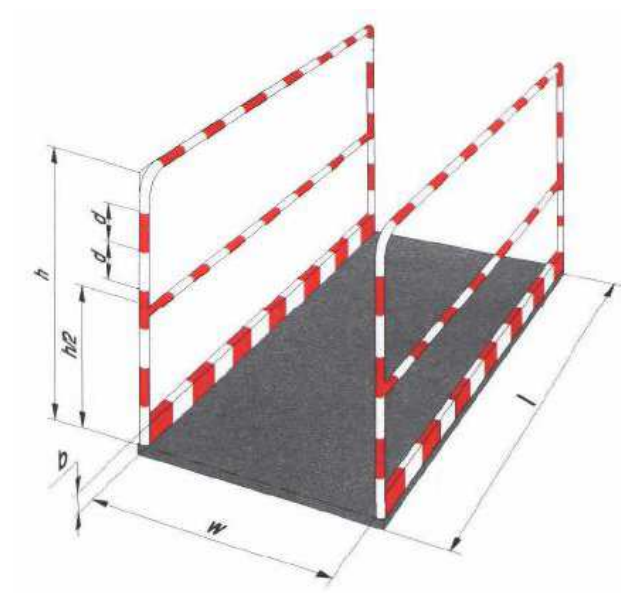
Rys. 22. Kładka dla pieszych U-28
