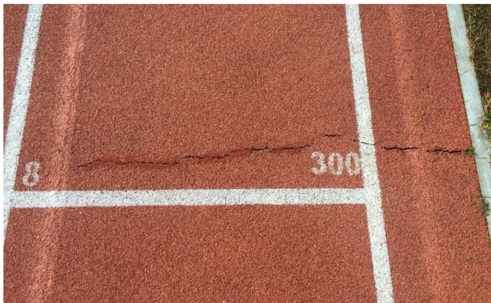
Fot. Spękania nawierzchni poliuretanowej - bieżnia okólna
