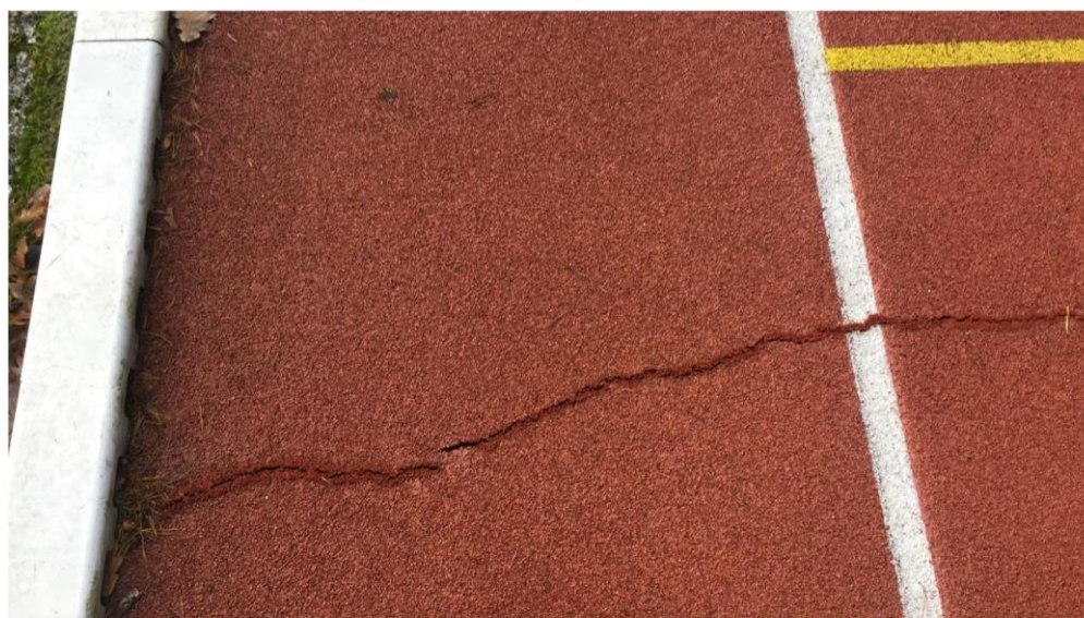
Fot. Spękania nawierzchni poliuretanowej - bieżnia okólna
