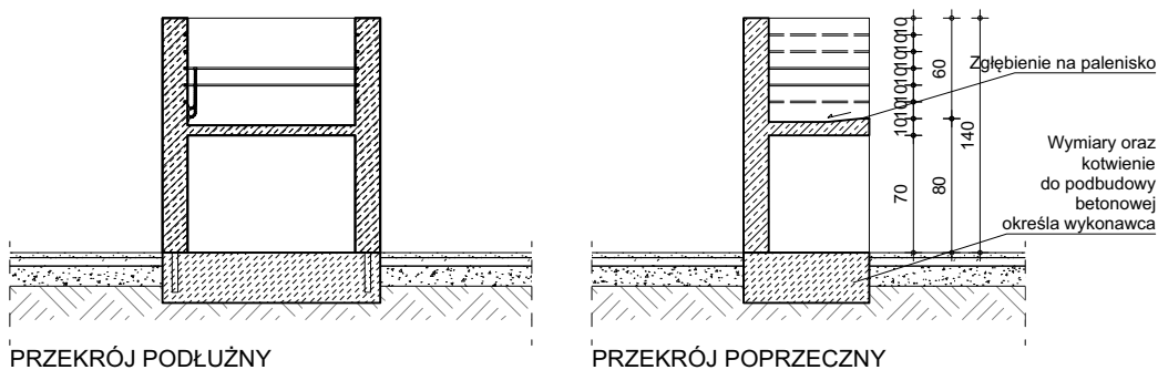
PRZEKRÓJ PODŁUŻNY
