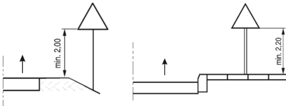
Rys. 1. Odległość znaków pionowych od krawędzi jezdni
