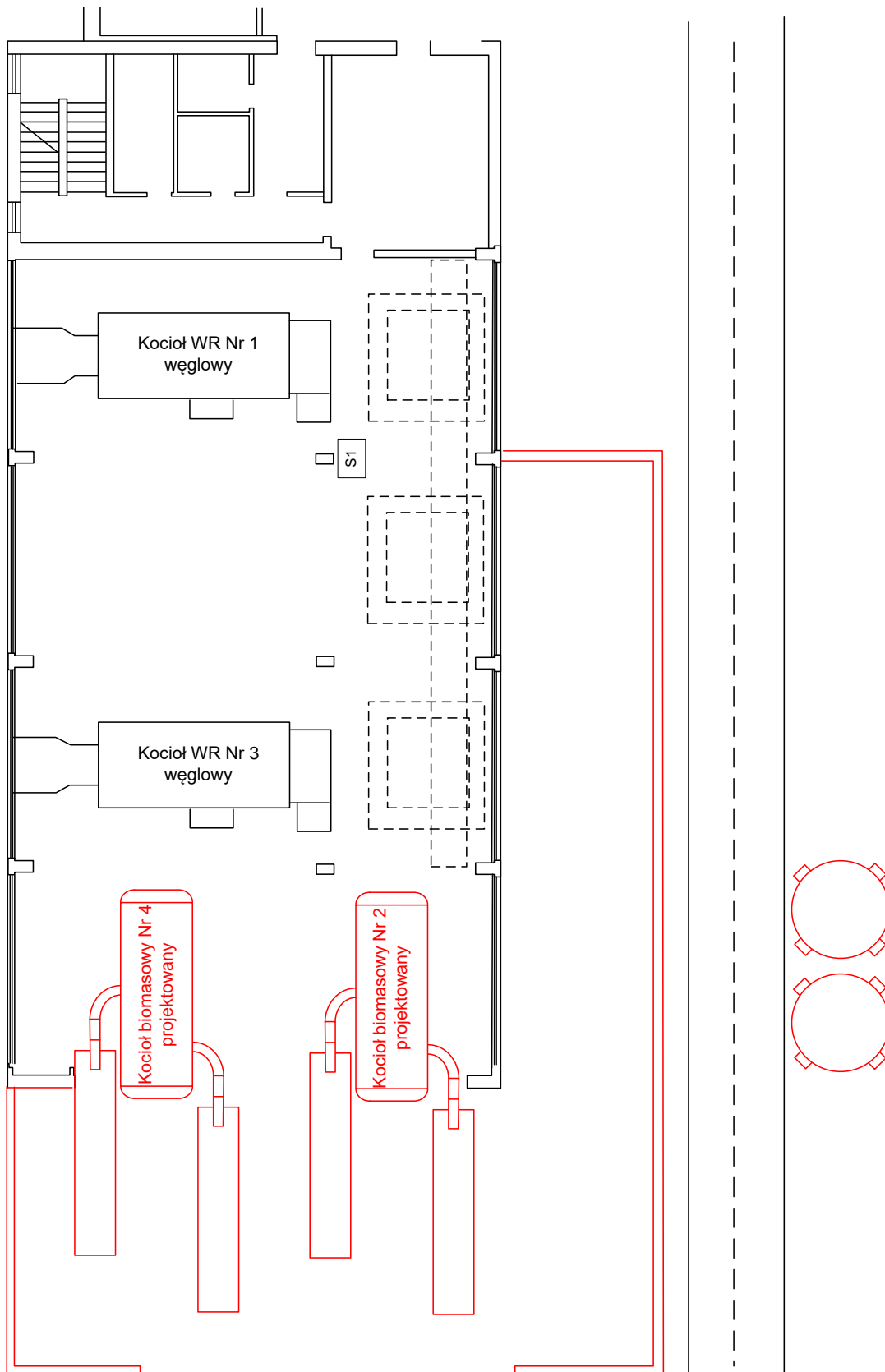
Rysunek 3 – wstępna koncepcja usytuowania podstawowych urządzeń
