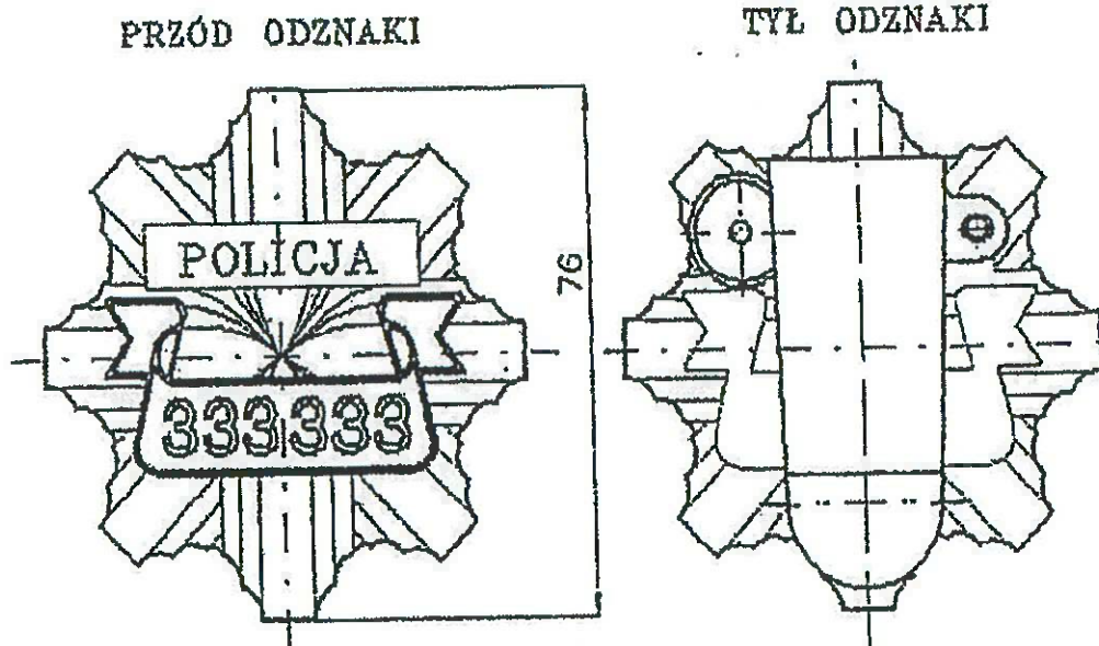
rys. Widok poglądowy odznaki identyfikacji indywidualnej policjanta.
