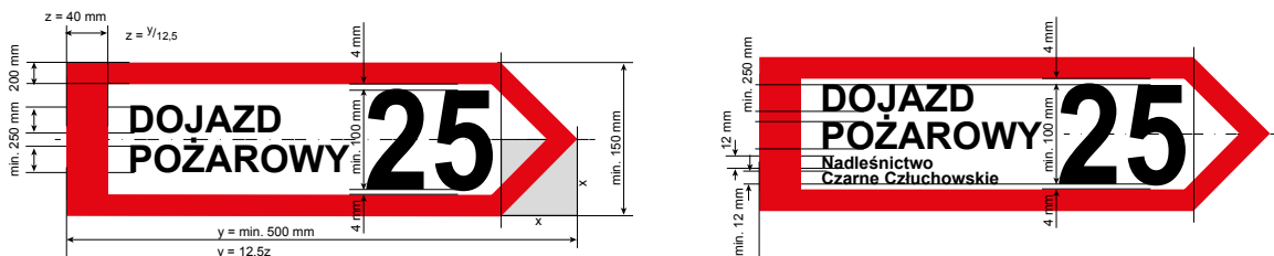
Tablice kierunkowe dojazdu pożarowego montowane na słupkach – wymiary minimalne.
