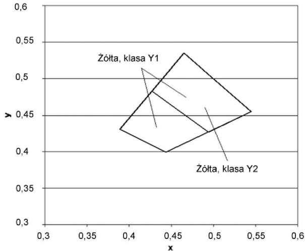
Rys.2. Współrzędne chromatyczości x,y dla barwy żółtej oznakowania
