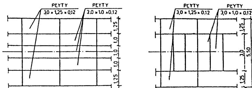
Rys. 3. Schemat układania płyt na drogach dojazdowych o dwóch pasach ruchu Sposób ułożenia płyt powinien być zgodny z dokumentacją projektową, SST lub wskazaniami Inżyniera.
