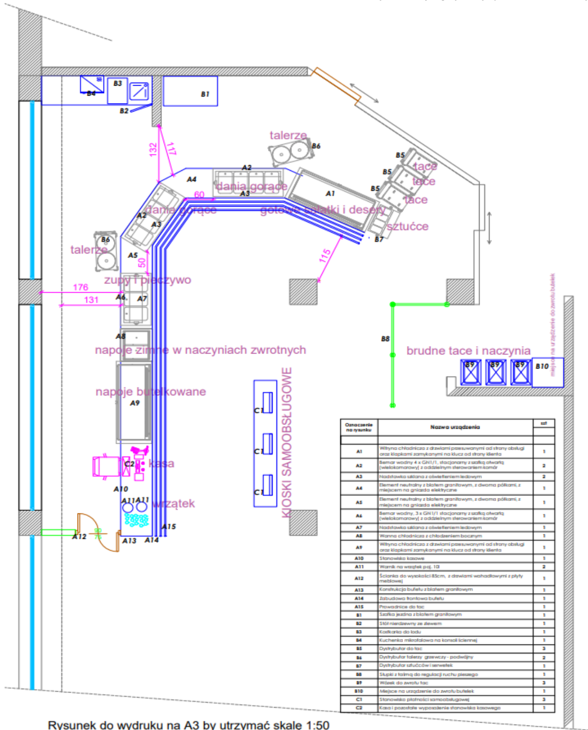
Rysunek do wydruku na A3 by utrzymać skalę 1:50
