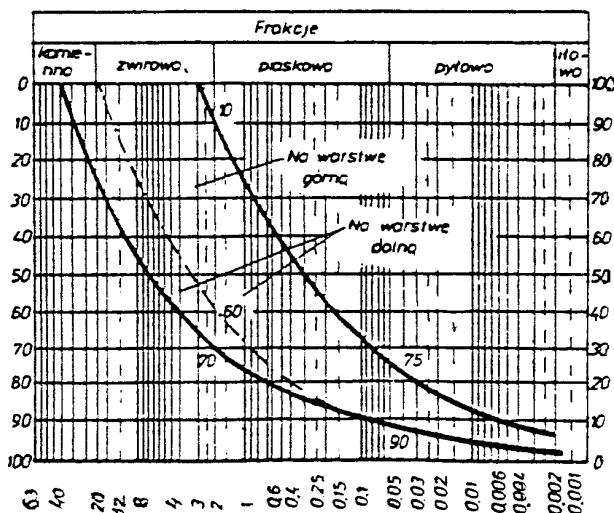
Rysunek 2. Obszar uziarnienia optymalnych mieszanek gliniasto-żwirowych
