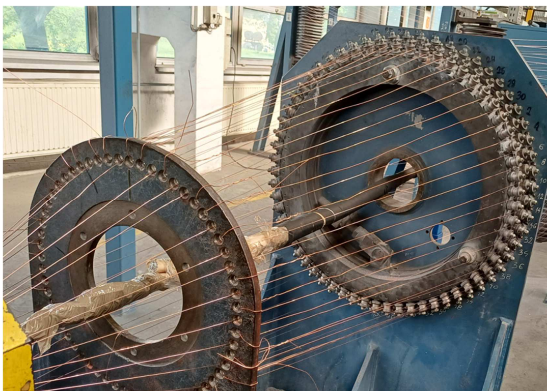
Zdj.2 (zestawienie podzielnicy obecnie na maszynie)
