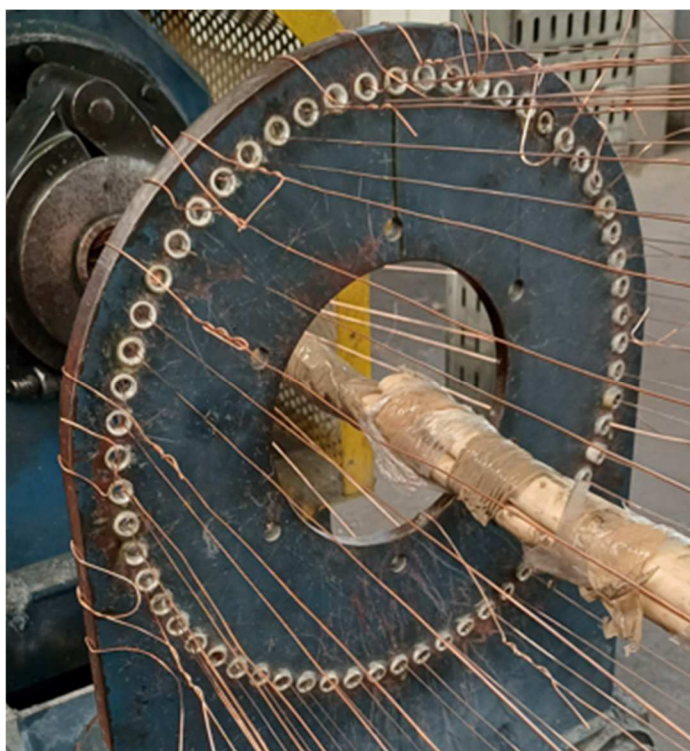
Zdj.2 (zestawienie podzielnicy obecnie na maszynie)
