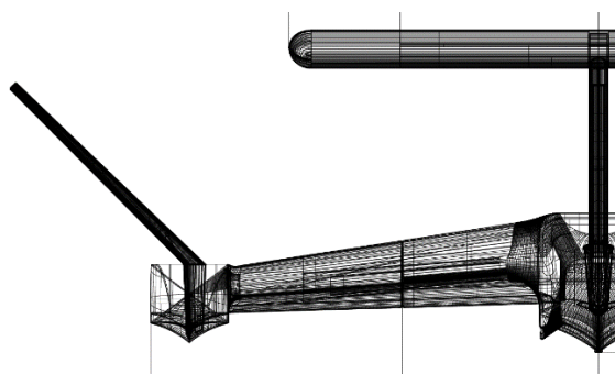
Rys.2c. Schemat geometrii obiektu – rzut wręgowy.
