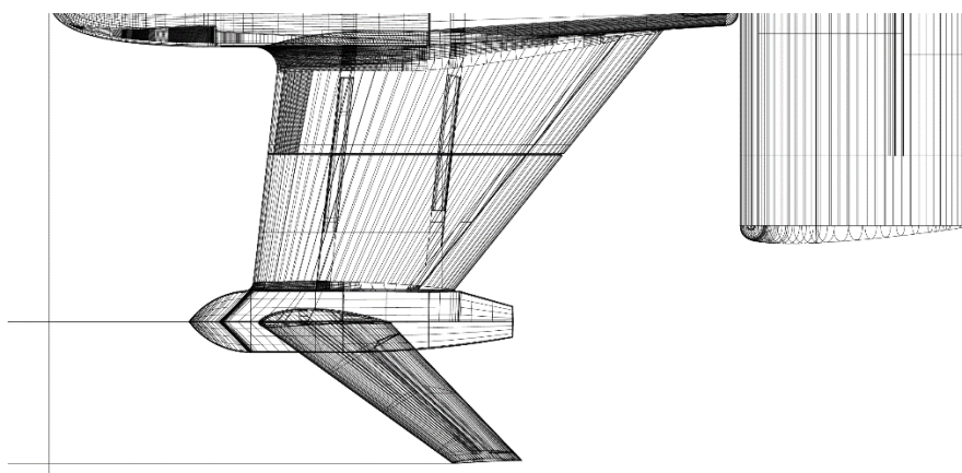
Rys.2b. Schemat geometrii obiektu – rzut wodnicowy.
