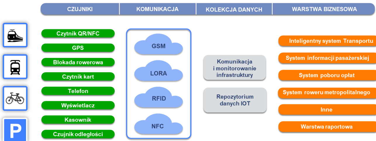
Rysunek 6 Architektura IoT
