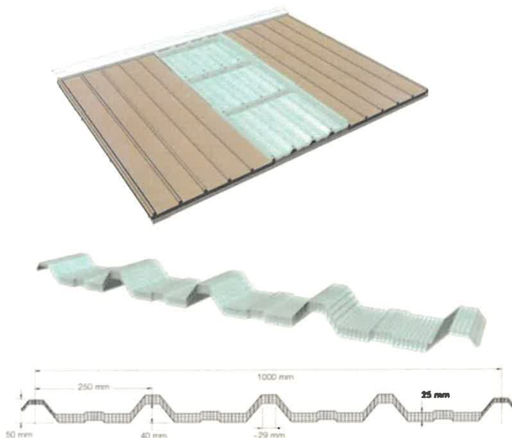
Rysunek 1 Świetlik dachowy, źródło: https://alfapanel.com.pl/pl/p/Swietlik-ALFA-ROOF-25040-20mm/571
