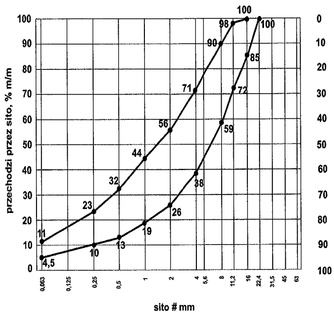
Rys. 4. Krzywe graniczne uziarnienia mieszanki mineralnej 0/16 mm
