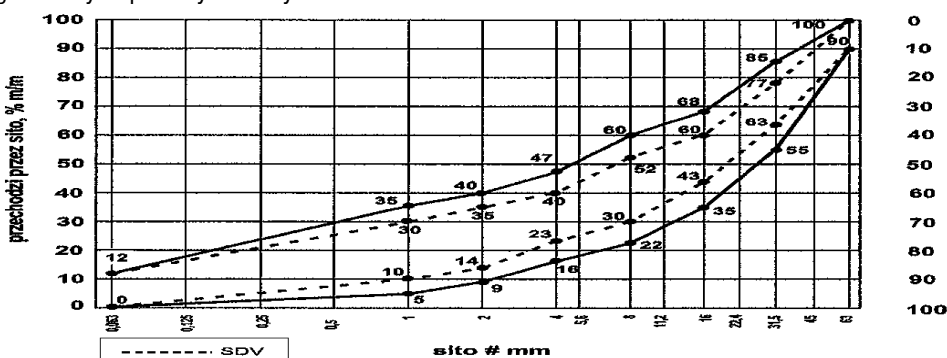
Rys. 1. Krzywe graniczne uziarnienia mieszanki kruszywa niezwiązanego 0/63 mm do warstw podbudowy pomocniczej
