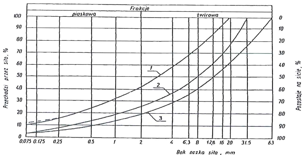
Rysunek 1. Pole dobrego uziarnienia kruszyw przeznaczonych na podbudowy
