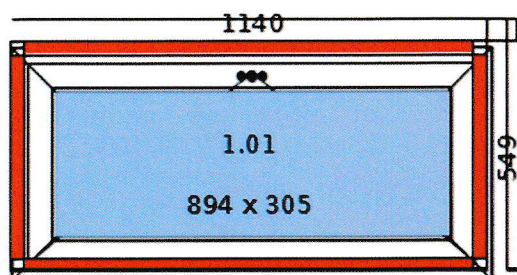
Widok wewnętrzny
