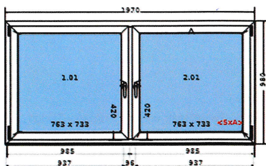
Widok wewnętrzny
