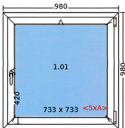
Widok wewnętrzny
