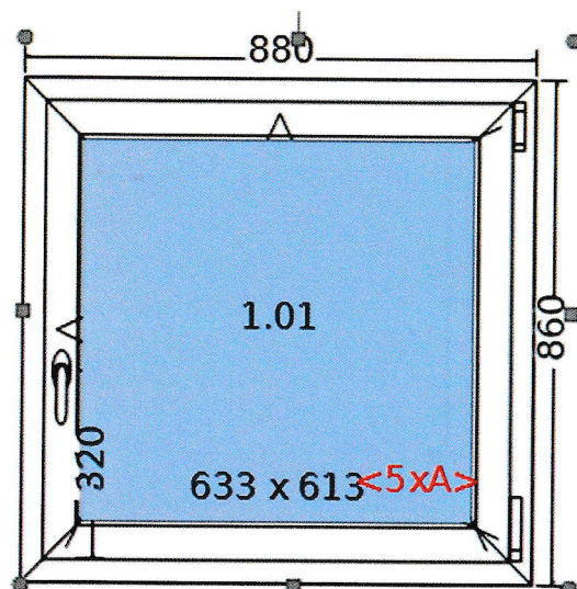
Widok wewnętrzny
