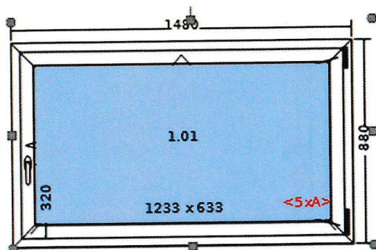
Widok wewnętrzny
