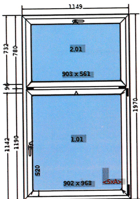
Widok wewnętrzny
