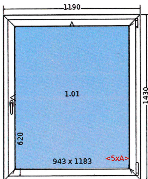
Widok wewnętrzny
