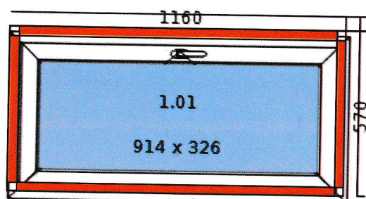
Widok wewnętrzny
