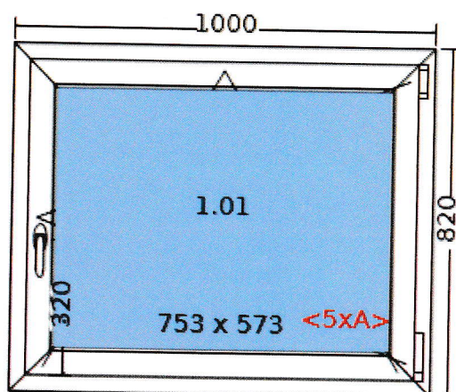
Widok wewnętrzny
