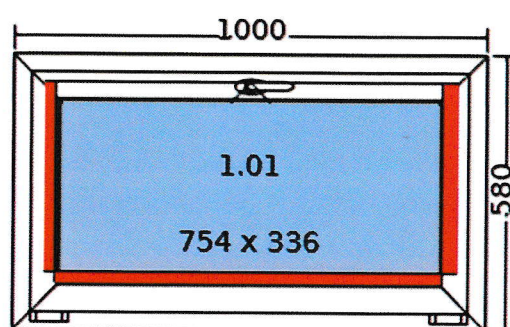
Widok wewnętrzny
