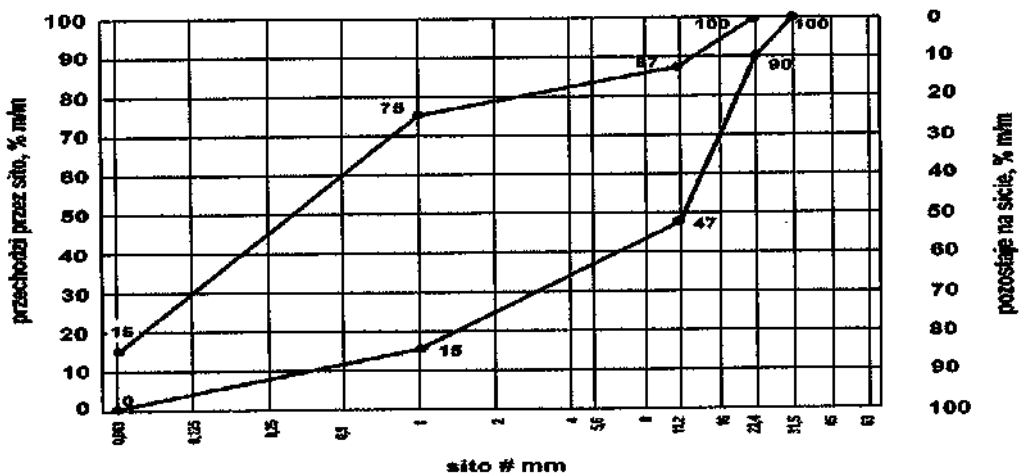
Rys. 4. Krzywe graniczne uziarnienia mieszanki kruszywa niezwiązanego 0/22,4 mm do warstw ulepszonego podłoża
