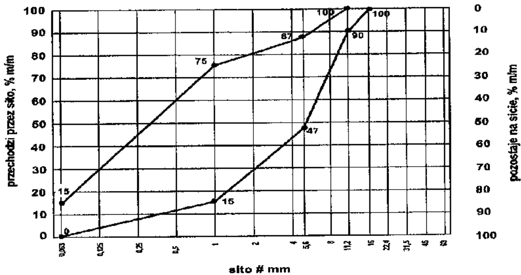
Rys. 2. Krzywe graniczne uziarnienia mieszanki kruszywa niezwiązanego 0/11,2 mm do warstw ulepszonego podłoża
