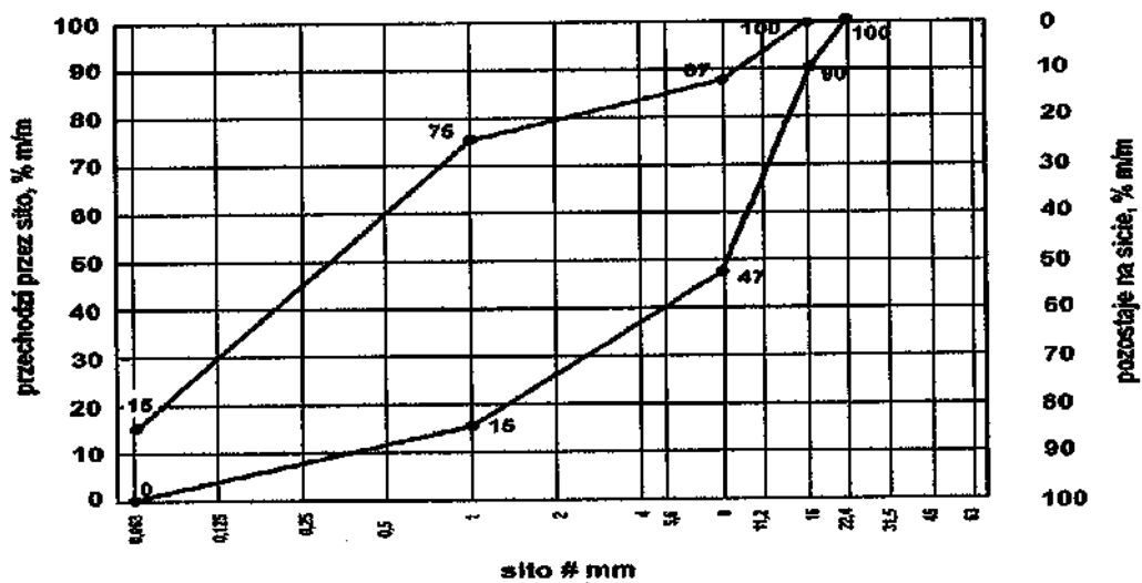
Rys. 3. Krzywe graniczne uziarnienia mieszanki kruszywa niezwiązanego 0/16 mm do warstw ulepszonego podłoża
