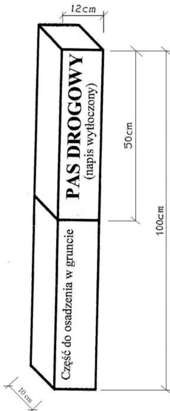
Rys. 1 Świadek punktu granicznego, pomalowany na żółto z czarnym napisem, wykonany z betonu B-25 zbrojonego 4 prętami \text{Ø}10
