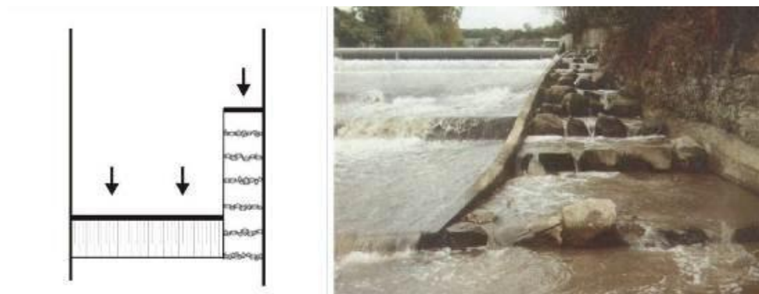
Przeławka kaskadowa przy budowlu hydrotechnicznej. (Jelonek 2008)
