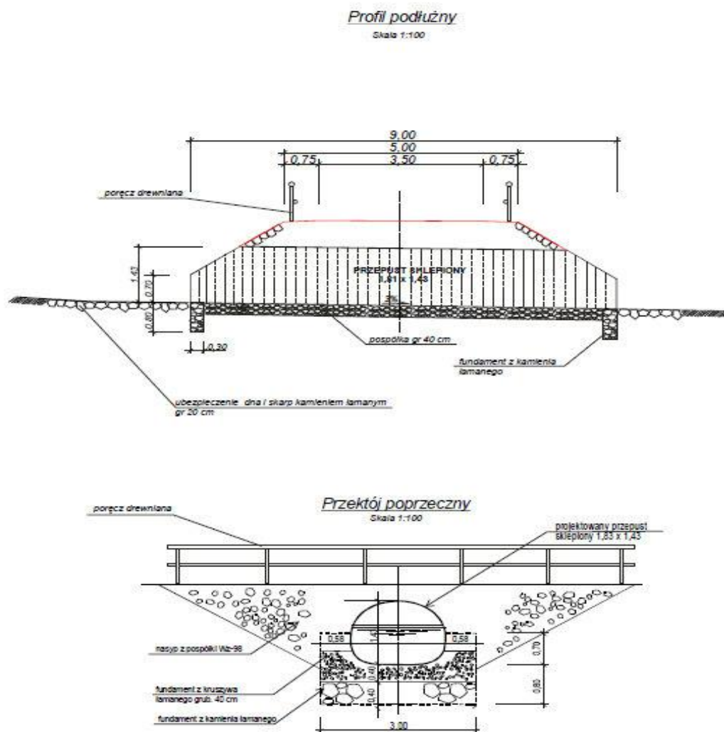
Rysunek brodu z Nadleśnictwa Łosie (RDLP Kraków)
