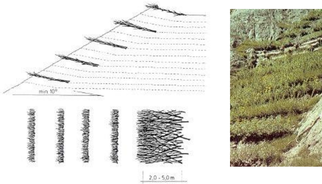
Krzewiaste umocnienia tarasowe na skarpie/osuwisku (Begemann i Schiechl 1999)
