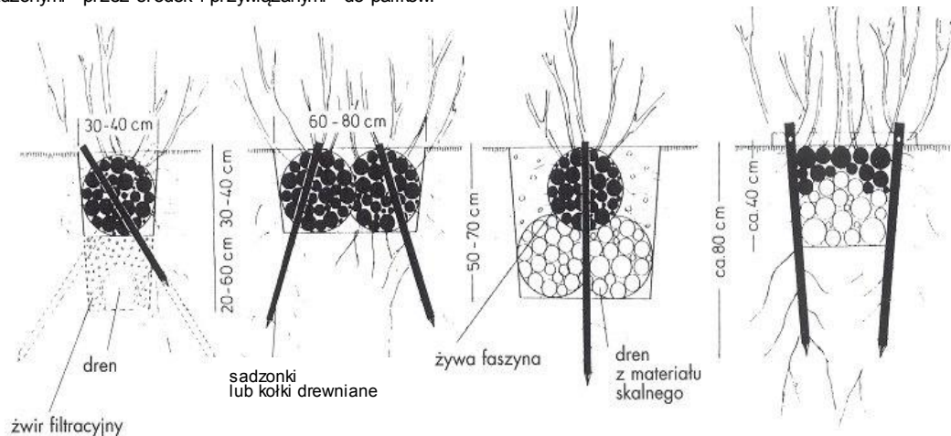
Różne rodzaje drenów faszynowych (Schiechtl 1973)
