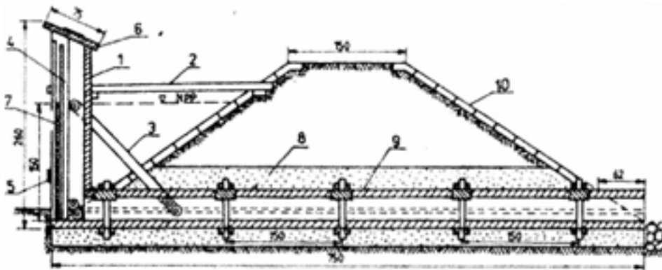
Mnich drewniany, piętrzenie 1,5m, światło 30x60cm (Mioduszewski 2003):
