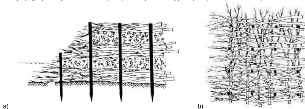
Brzegosłon krzyżowy a - przekrój poprzeczny, b – rzut z góry (Begemann i Schiechtl 1999)
