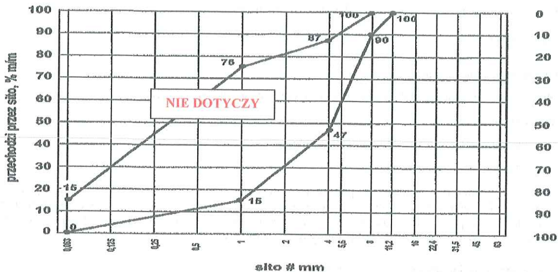
Rys. 1. Krzywe graniczne uziarnienia mieszanki kruszywa niezwiązanego 0/4 mm do nawierzchni
