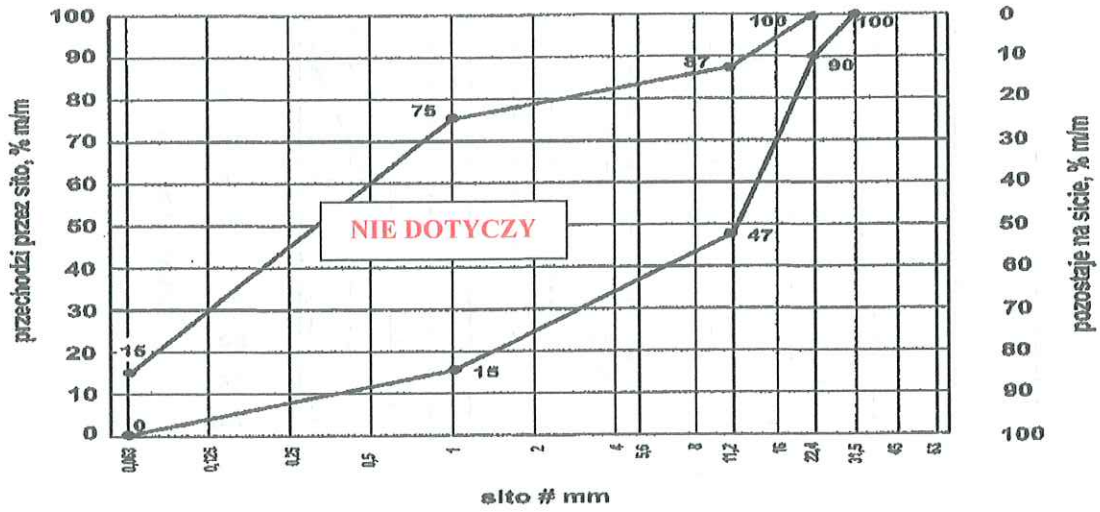
Rys. 4. Krzywe graniczne uziarnienia mieszanki kruszywa niezwiązanego 0/22,5 mm do nawierzchni
