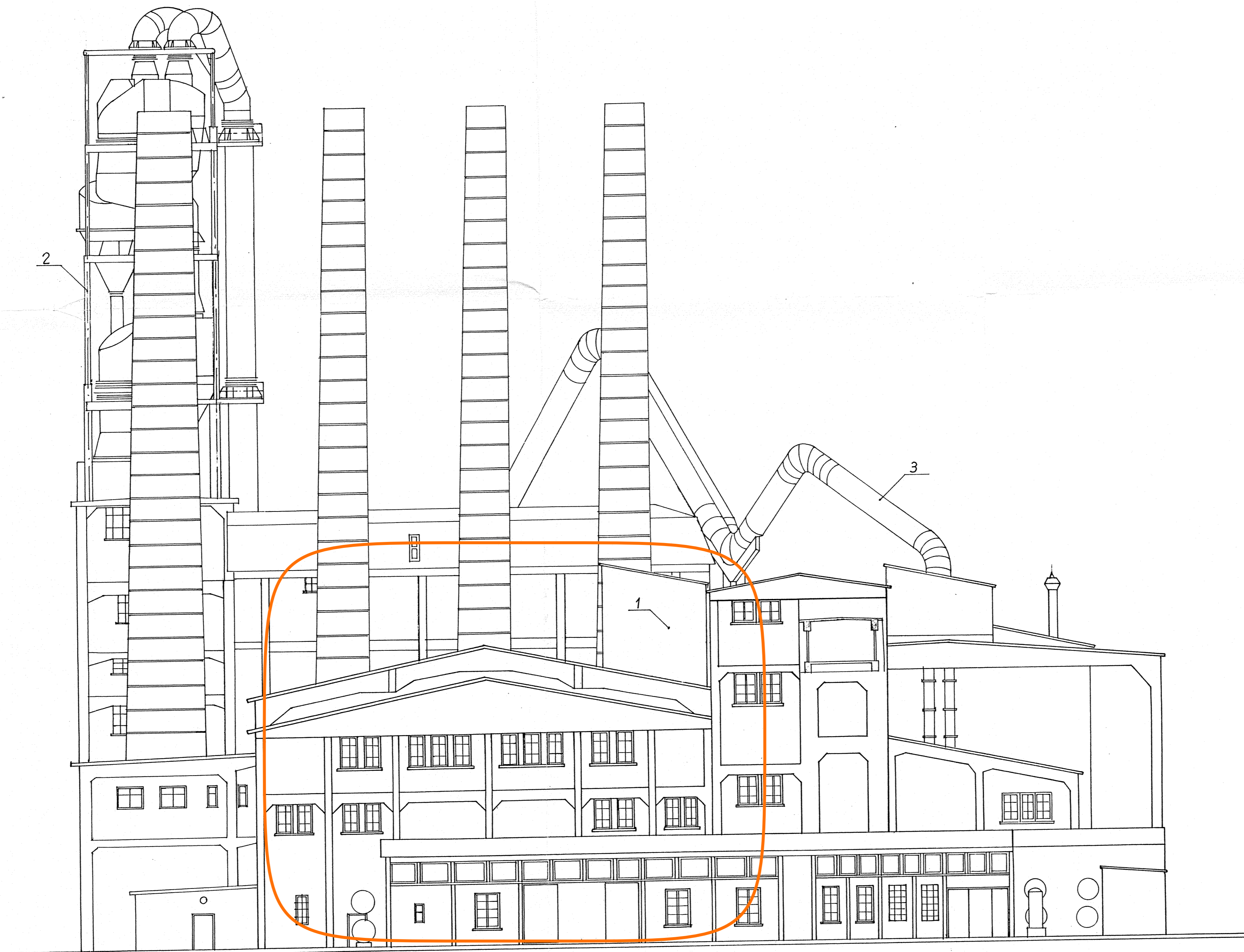
ELEWACJA ZACHODNIA
