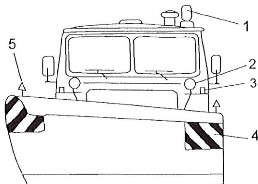
Rys. 3. Oznakowanie pluga i nośnika 1 – lampa ostrzegawcza barwy żółtej, 2 – reflektory samochodu podniesione na wspornikach, 3 – kierunkowskazy umieszczone na wspornikach, 4 – biało-czerwone odblaskowe pasy na końcach odkładnicy, 5 – lampa biała widoczna z przodu i czerwona widoczna z tyłu
