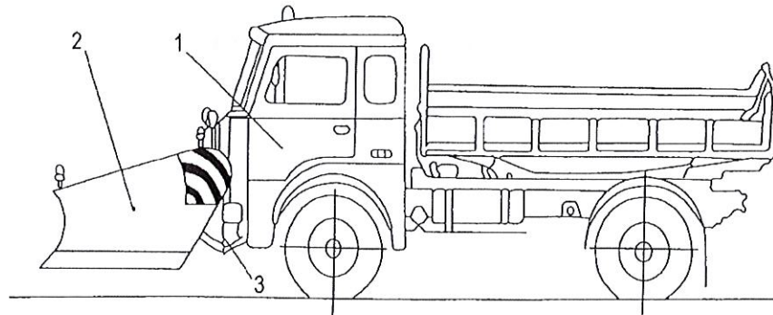
Rys. 2. Schemat pluga i czołownicy (widok z boku)
