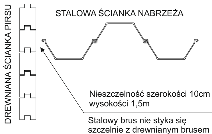
Rys. 1 Schemat występującej nieszczelności
