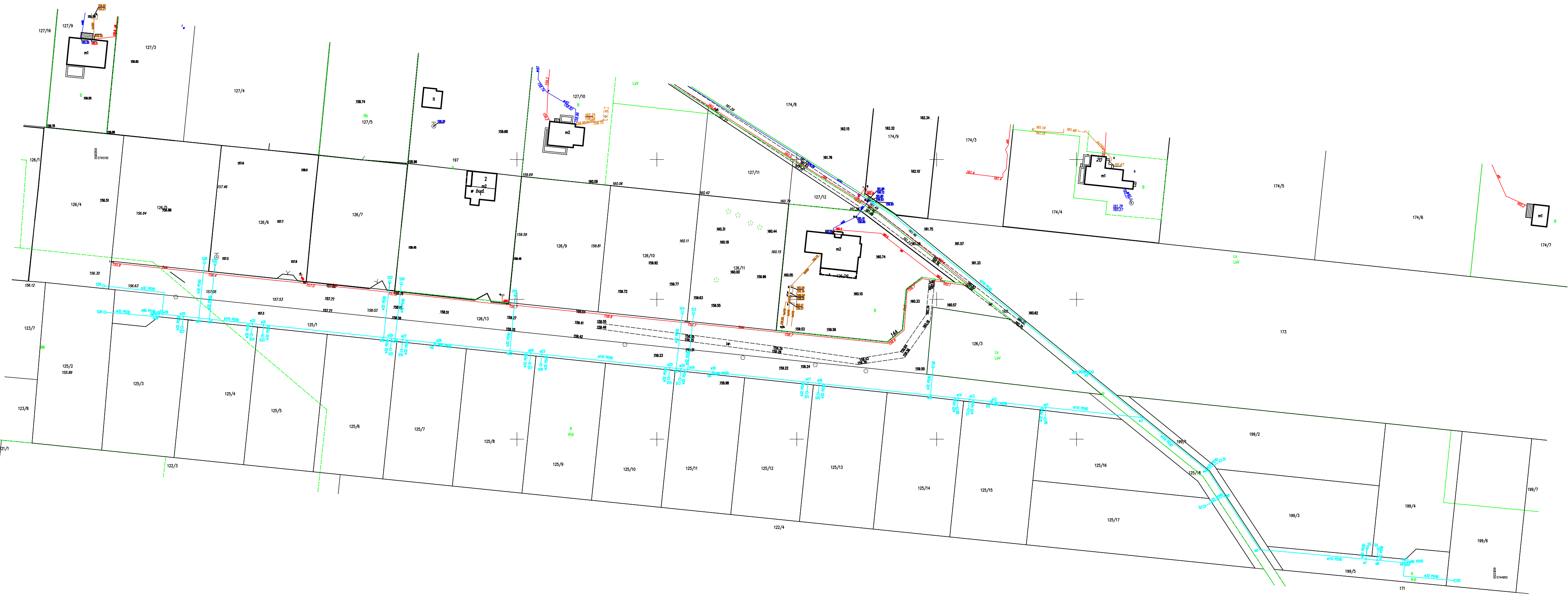
Mapa koncepcyjna budowy wodociągu i 29 przyłączy na dz. ewid. nr: 125/1, 125/2, 125/3, 125/4, 125/5, 125/6, 125/7, 125/8, 125/9, 125/10, 125/11, 125/12, 125/13, 125/14, 125/15, 125/16, 125/17, 125/18, 126/3, 126/4, 126/5, 126/7, 126/9, 126/10, 126/11, 126/13, 168, 199/1, 199/2, 199/3, 199/4, 199/5, 199/6. w obrębie Ciężków.
