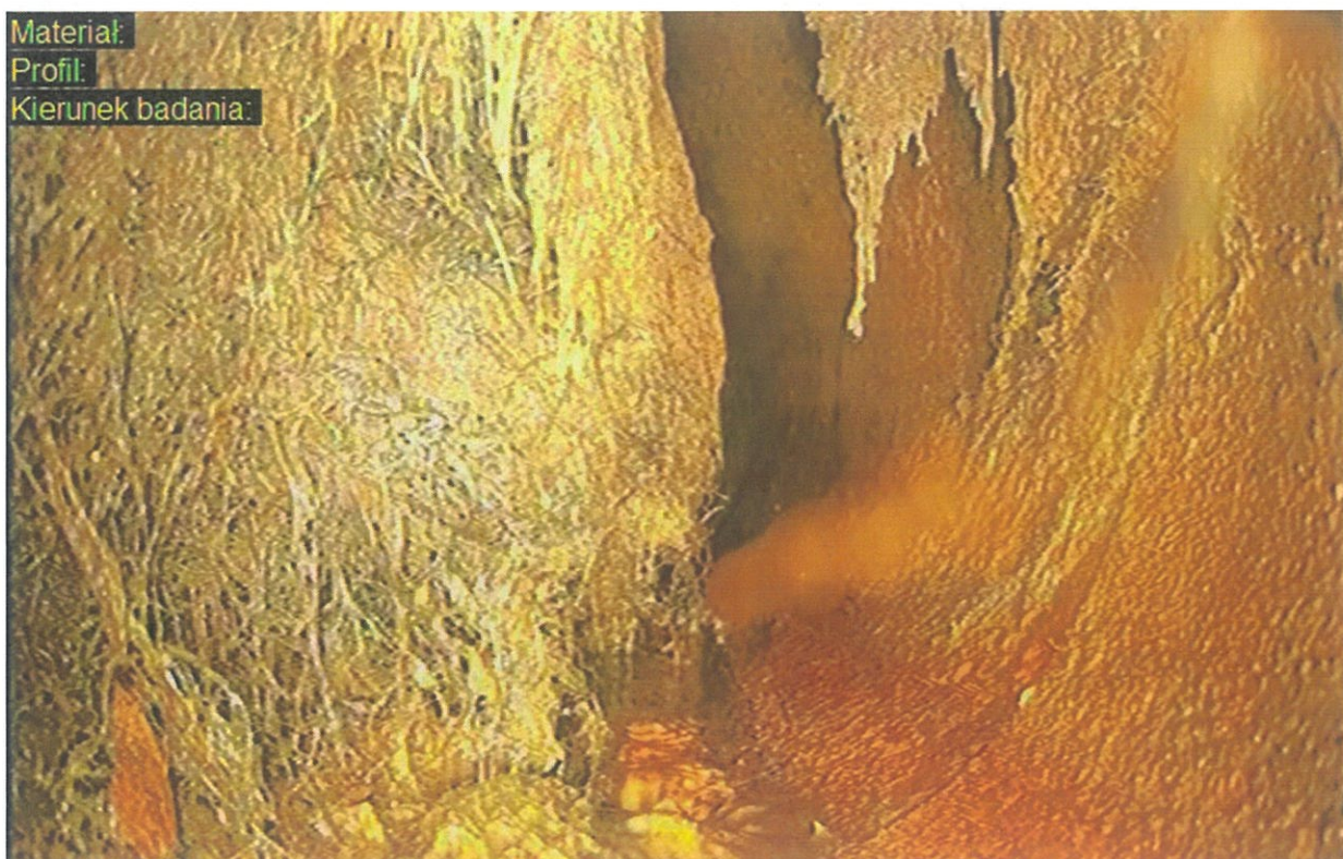
Fot. nr 6 widok stanu wnętrza rurociągu
