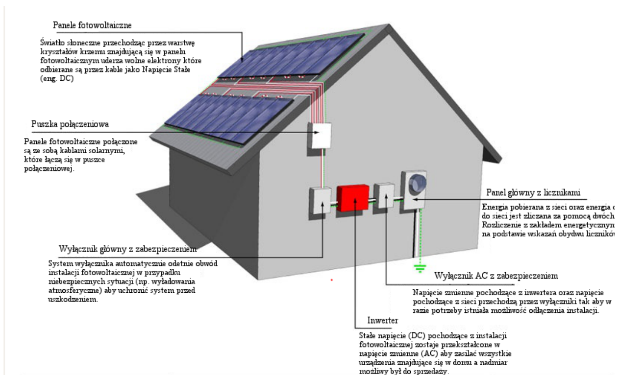
Rysunek 4 Sposób podłączenia instalacji do sieci
