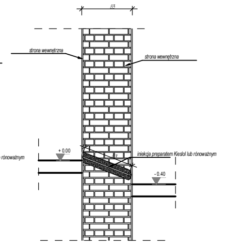
SZCZEGÓŁ e - e
