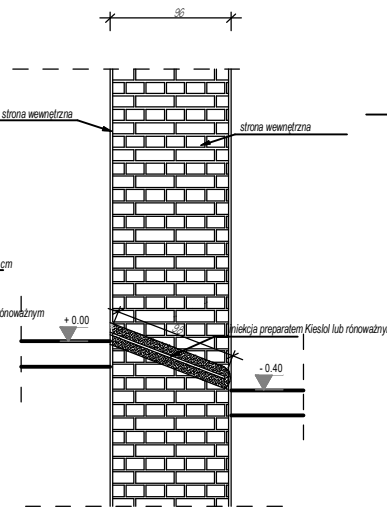
SZCZEGÓŁ d - d
