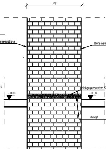
SZCZEGÓŁ b - b
