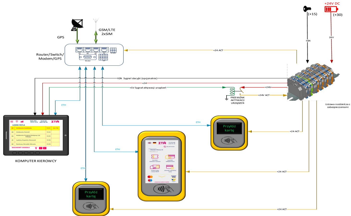
Załącznik 1: Schemat ideowy instalacji wariant „METROLINIA”
