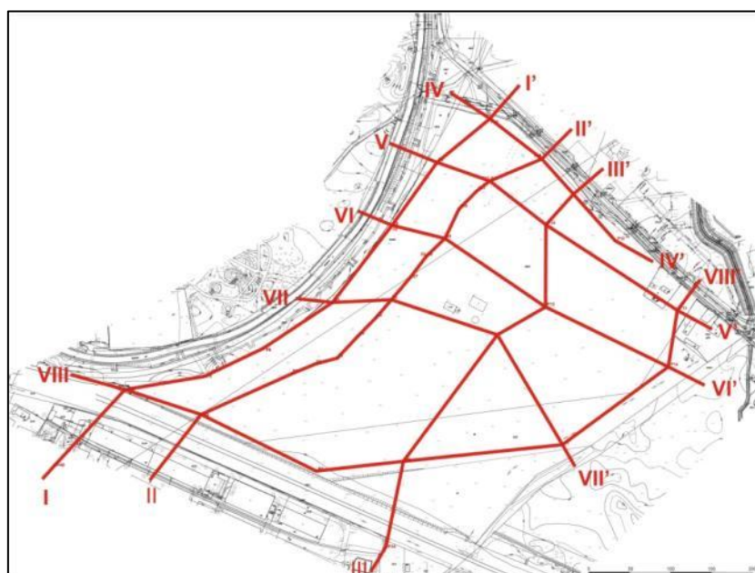
Fig. 18. Linie przekrojów geologicznych wykonanych dla potrzeb interpretacji warunków hydrogeologicznych
