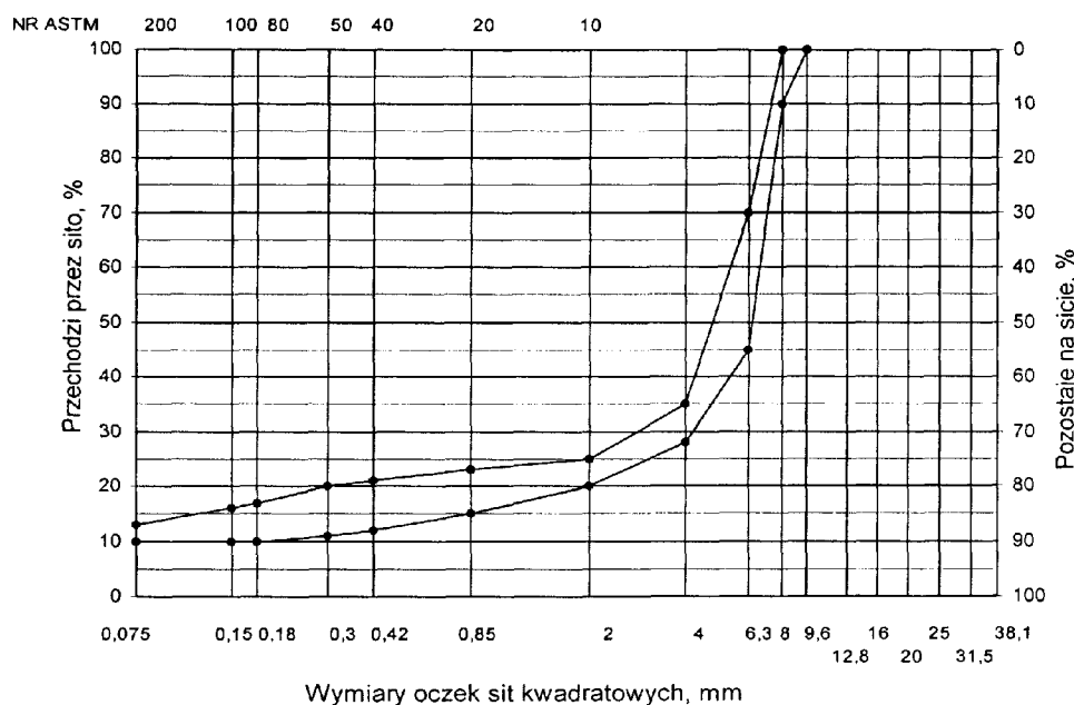
Rys. 7. Krzywe graniczne uziarnienia mieszanki mineralnej SMA od 0 do 8 mm do warstwy ściernalnej nawierzchni drogi o obciążeniu ruchem od KR3 do KR6
