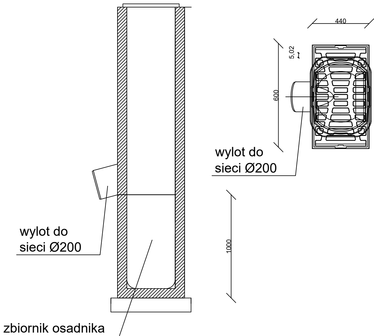
PRZEKROJ A
