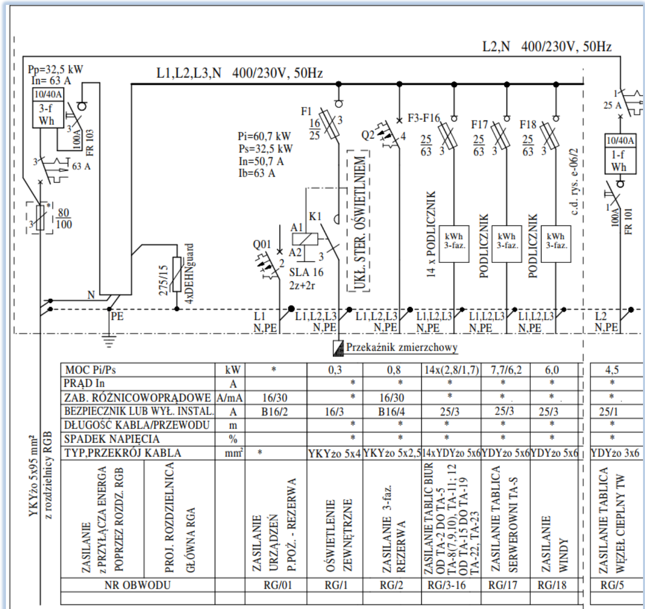
Rysunek nr 11. Miejsce adaptacji -podłączenia przewodu AC w rozdzielnicy głównej obiektu. Wykożystac pole rezerwowe nr 3-RG/2.
