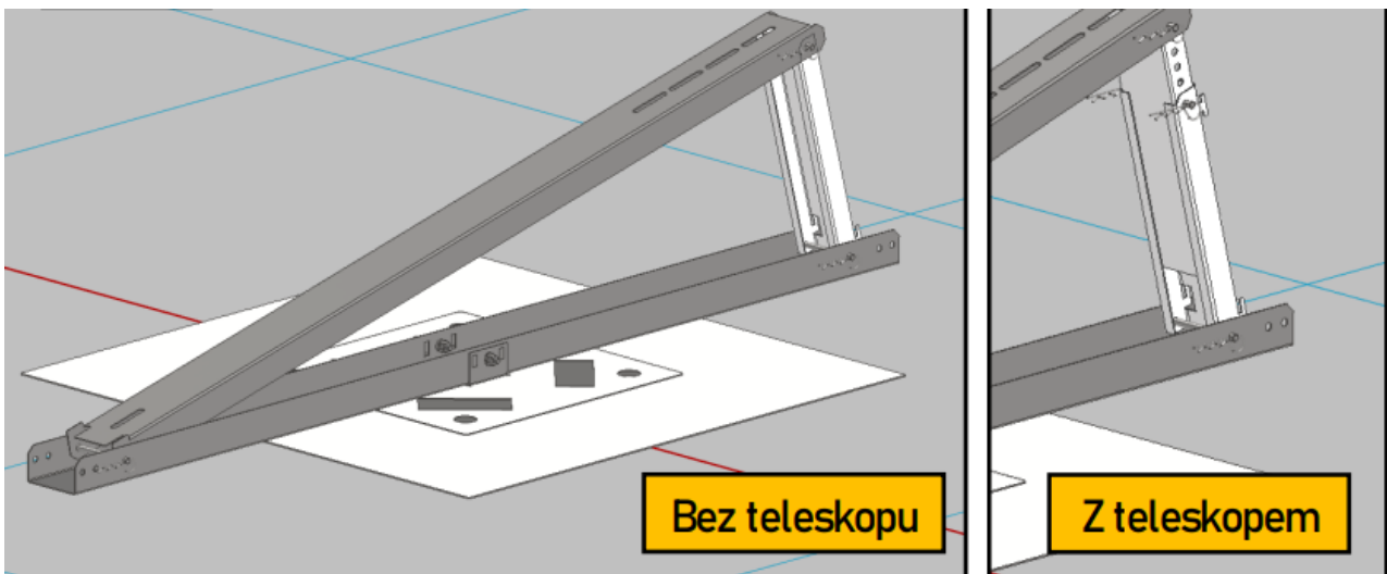
Zdjęcie nr 6. Przykładowy widok systemu mocowania konstrukcji -zgrzewanej Wschód-Zachód.
