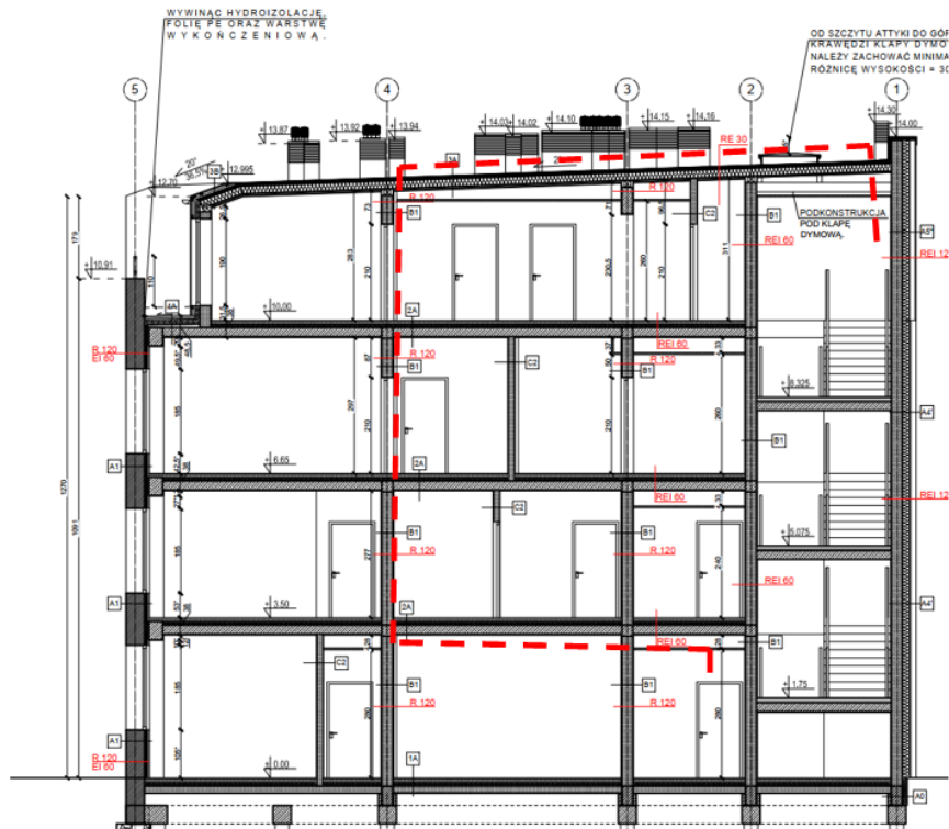
Rysunek nr 8. Przekrój poprzeczny. Widok trasy kablowej AC.
