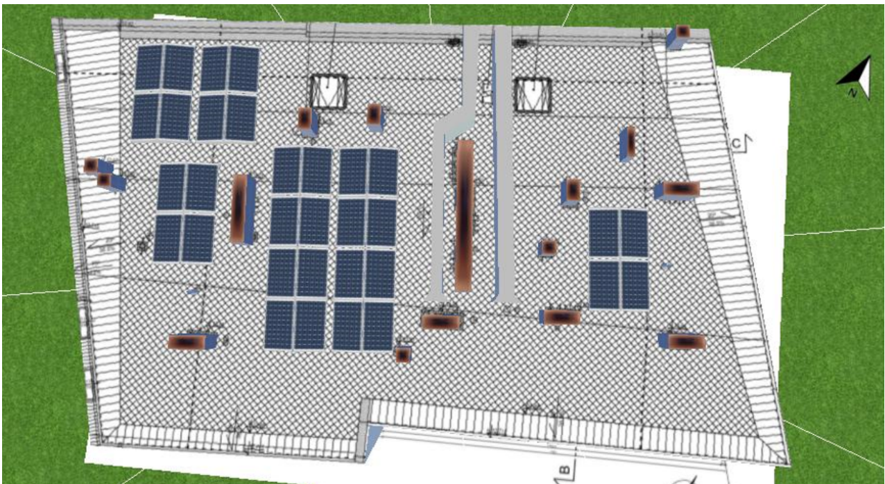
Rysunek 2: Umieszczenie generatora fotowoltaicznego i grupy przetwornic
