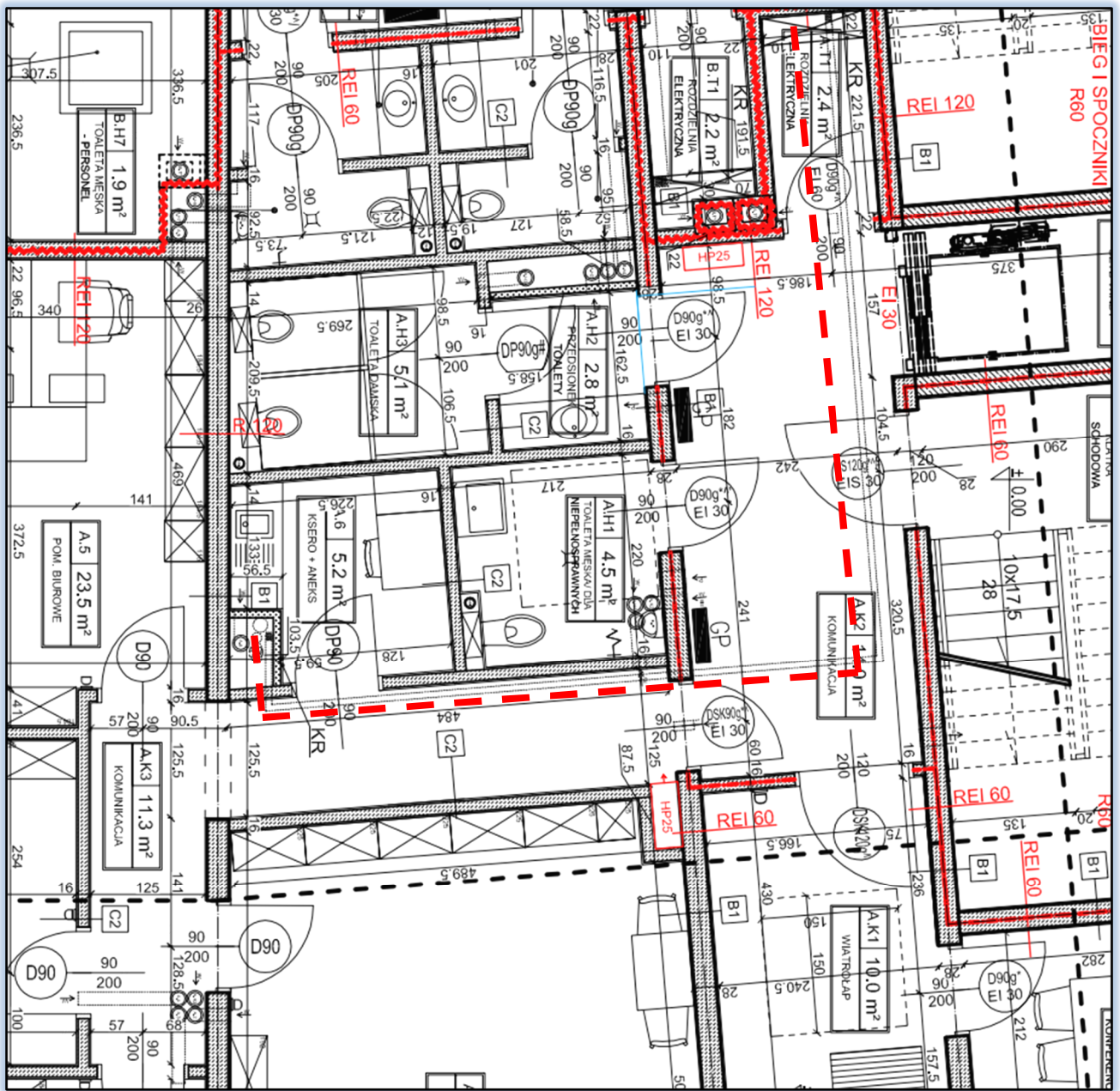
Rysunek nr 10. Miejsce wyprowadzenia kabla AC z szachtu kablowego. Przewód układać w przestrzeni nad sufitem podwieszanym na istniejących korytkach kablowych. Przewód ułożyć do rozdzielni głównej obiektu na parterze.
