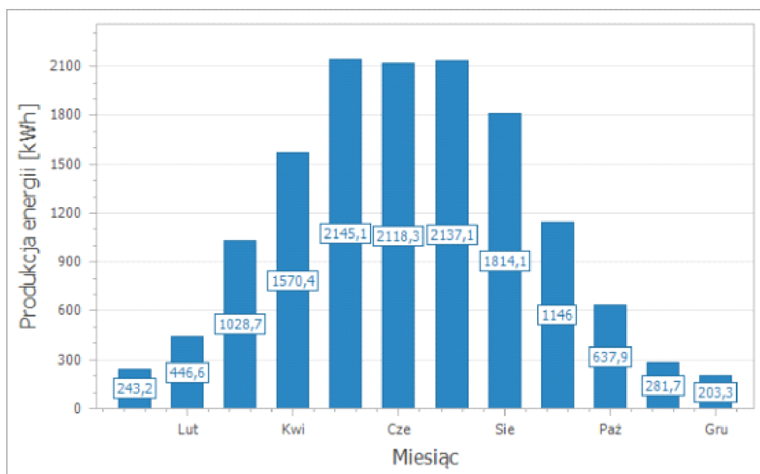
Rysunek nr 5. Produkcja energii
