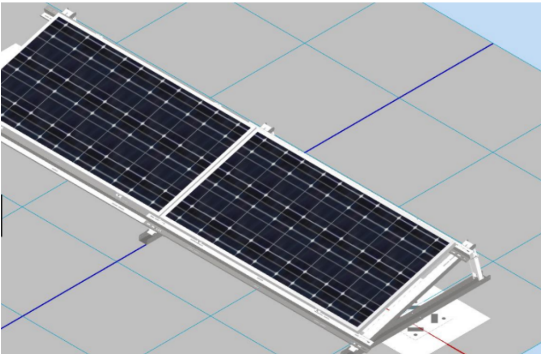
Rysunek nr 6. System konstrukcji - zgrzewany – bezbalastowy
