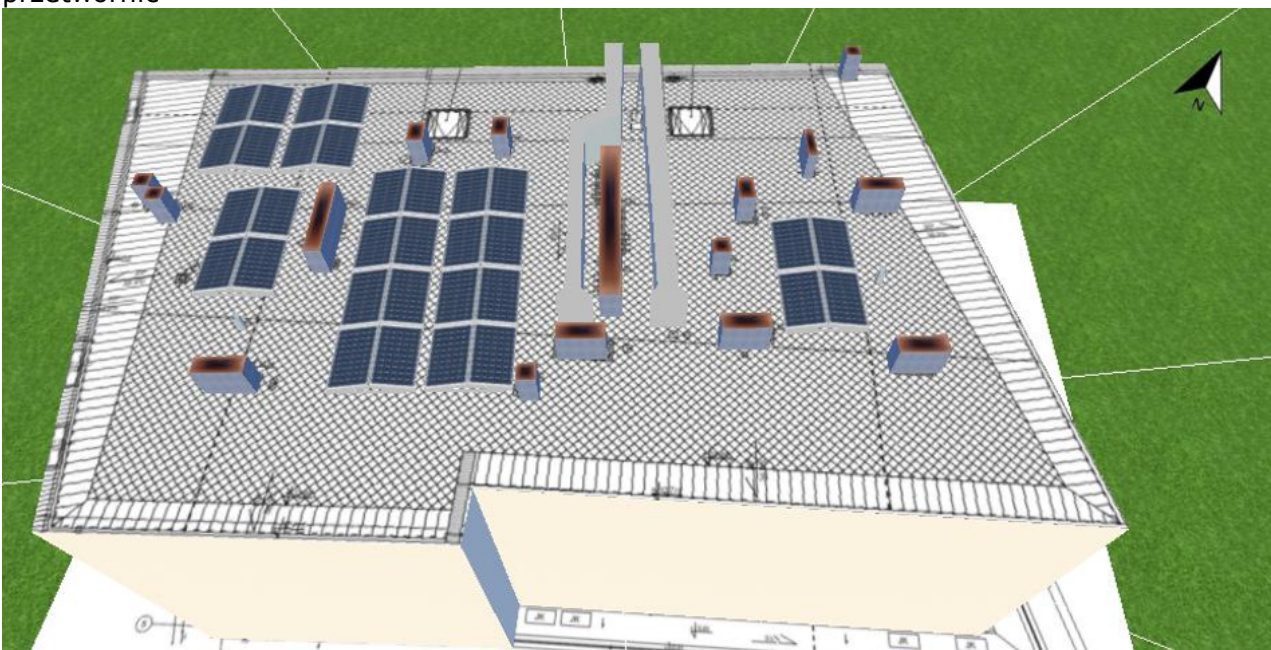
Rysunek 3: Realistyczny widok instalacji system
