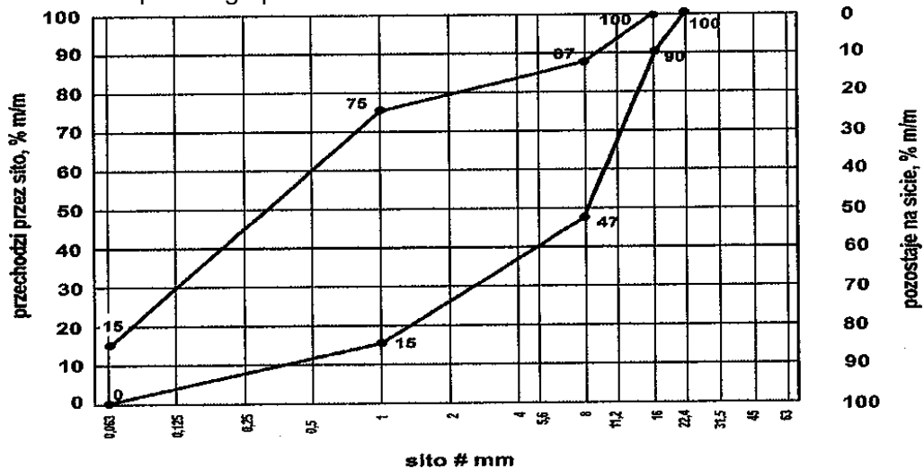
Rys. 3. Krzywe graniczne uziarnienia mieszanki kruszyw 0/16 mm do górnej warstwy ulepszonego podłoża
