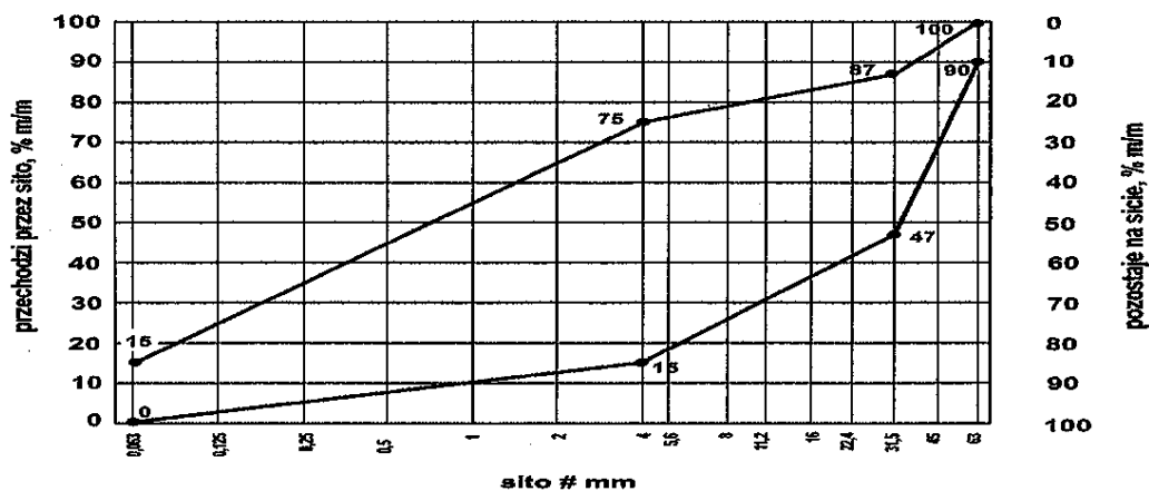
Rys. 7. Krzywe graniczne uziarnienia mieszanki kruszyw 0/63 mm do górnej warstwy ulepszanego podłoża
