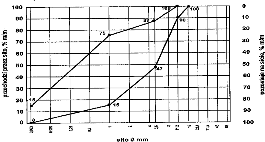
Rys. 2. Krzywe graniczne uziarnienia mieszanki kruszyw 0/11,2 mm do górnej warstwy ulepszonego podłoża
