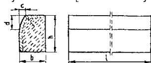
Wymiary krawężników, cm
