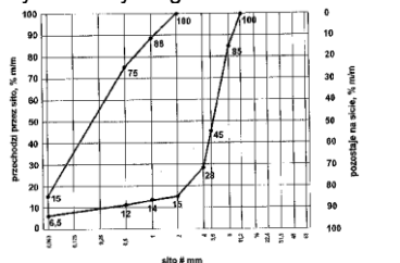
Rys. 5. Krzywe graniczne uziarnienia mieszanki mineralnej 0/8 mm
