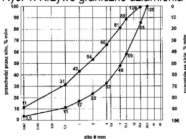
Rys. 2. Krzywe graniczne uziarnienia mieszanki mineralnej 0/22,4 mm
