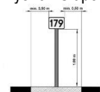
Rys. 4. Znak kilometrowy U-7 na samodzielnym słupku
