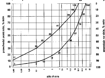
Rys. 1. Krzywe graniczne uziarnienia mieszanki mineralnej 0/31,5 mm
