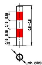
Rys. 5. Słupki blokujący U-12c
