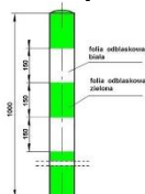
Rys. 3. Słupki krawędziowy U-2
