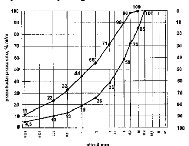
Rys. 3. Krzywe graniczne uziarnienia mieszanki mineralnej 0/16 mm
