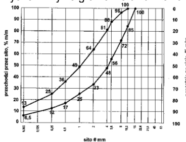
Rys. 4. Krzywe graniczne uziarnienia mieszanki mineralnej 0/11,2 mm
