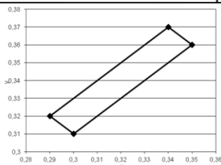
Rysunek 1 - Współrzędne chromatyczności x, y barwy białej
