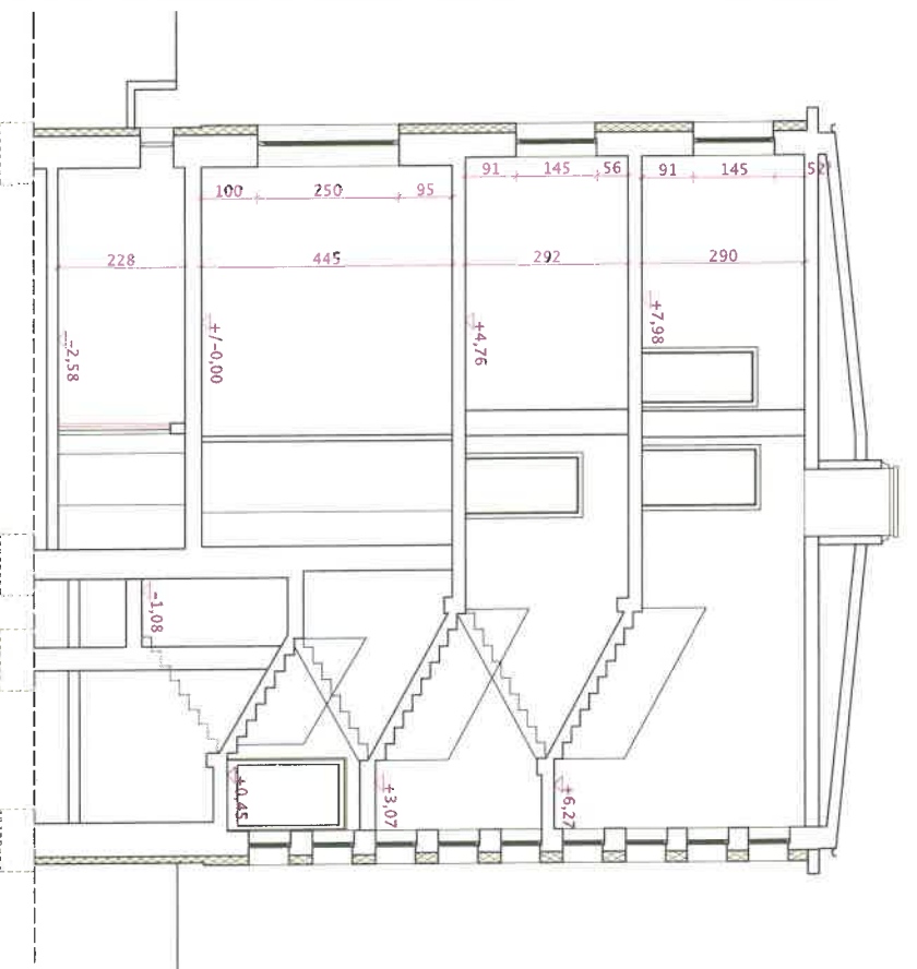
Przekrój B-B
