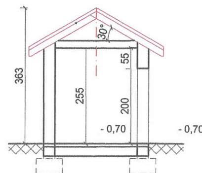
PRZEKRÓJ B-B skala 1:100
