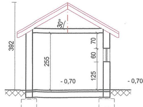
PRZEKRÓJ C-C skala 1:100
