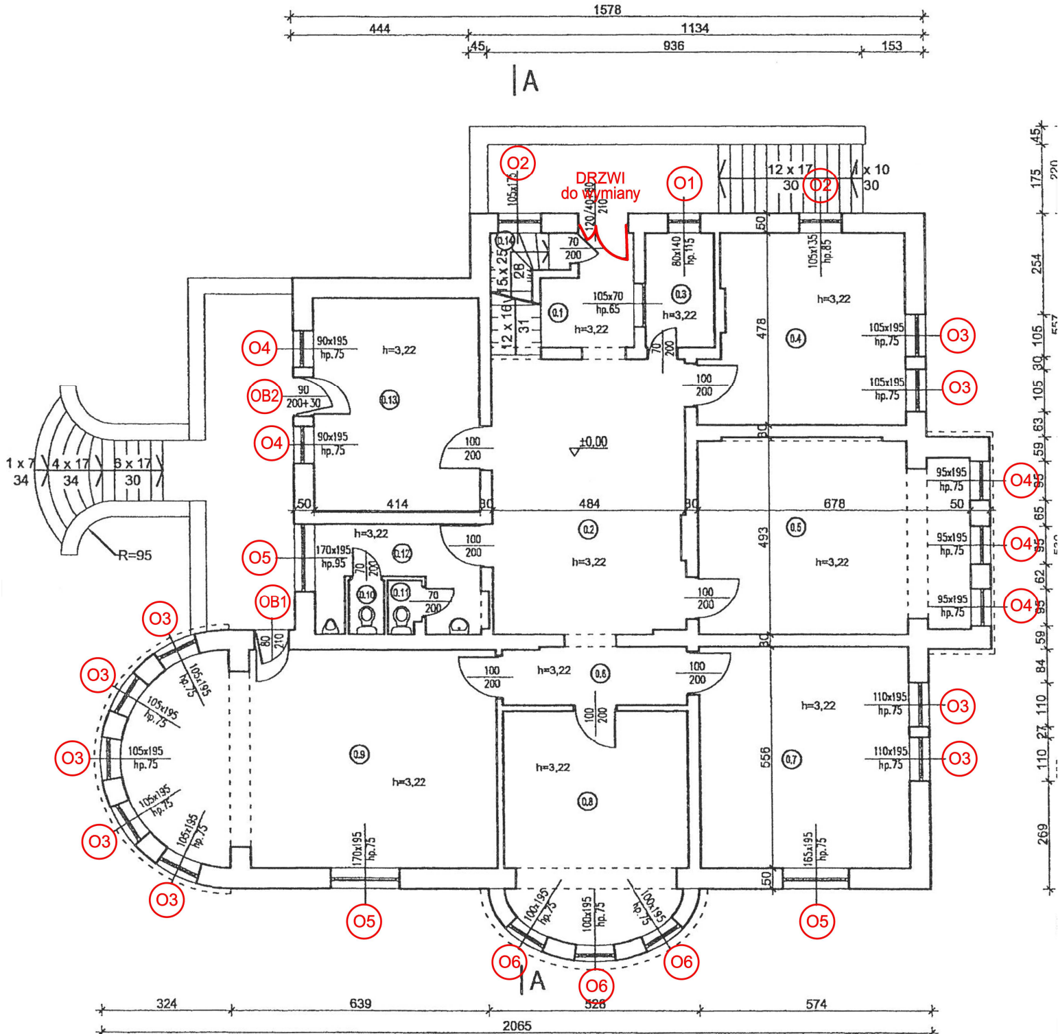
Rzut parteru
