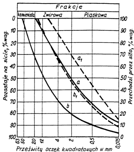
Rysunek 1. Obszar uziarnienia optymalnych mieszanek żwirowych
