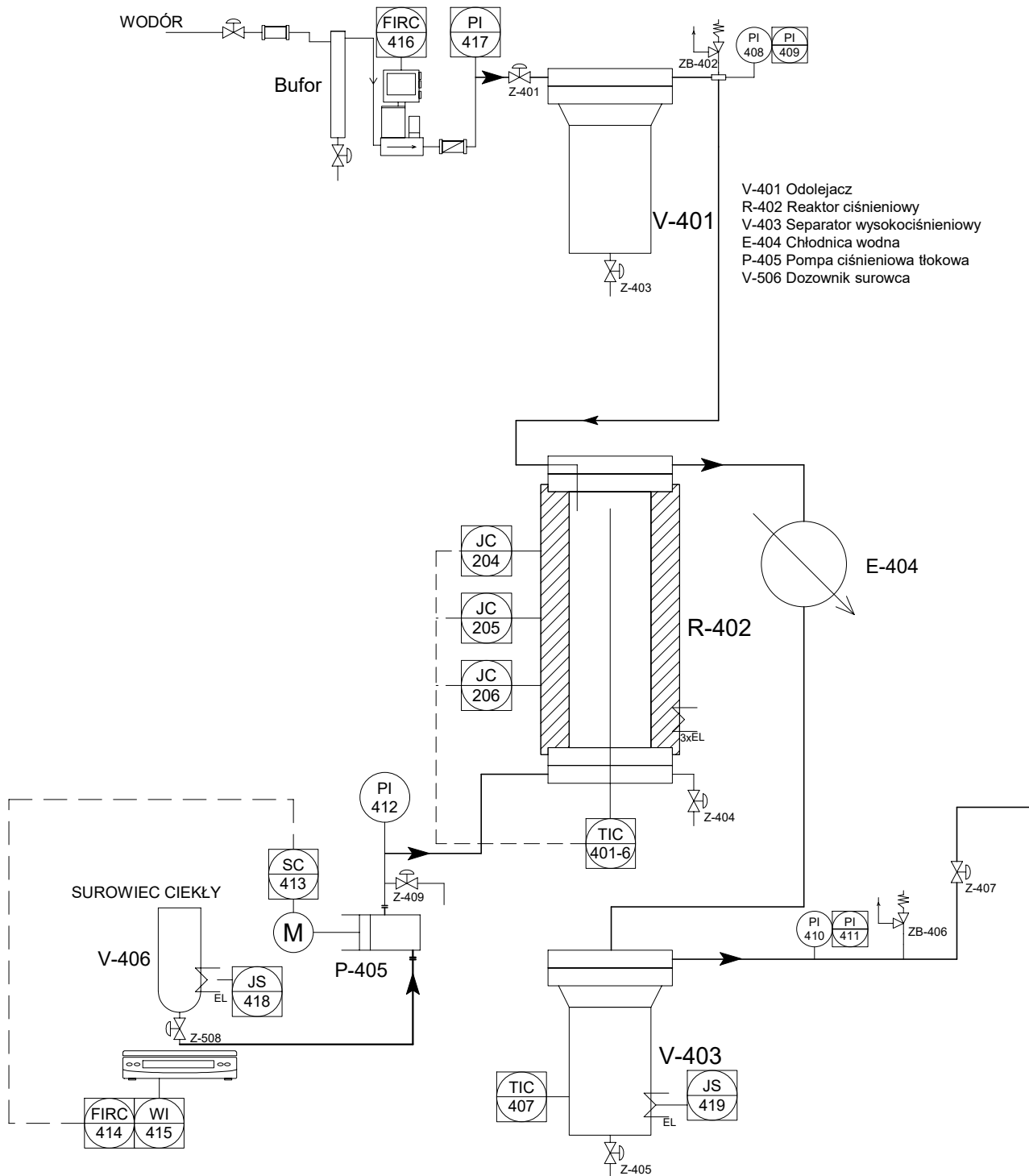
INSTALACJA LABORATORYJNA CIĄGŁA LAB-CON
