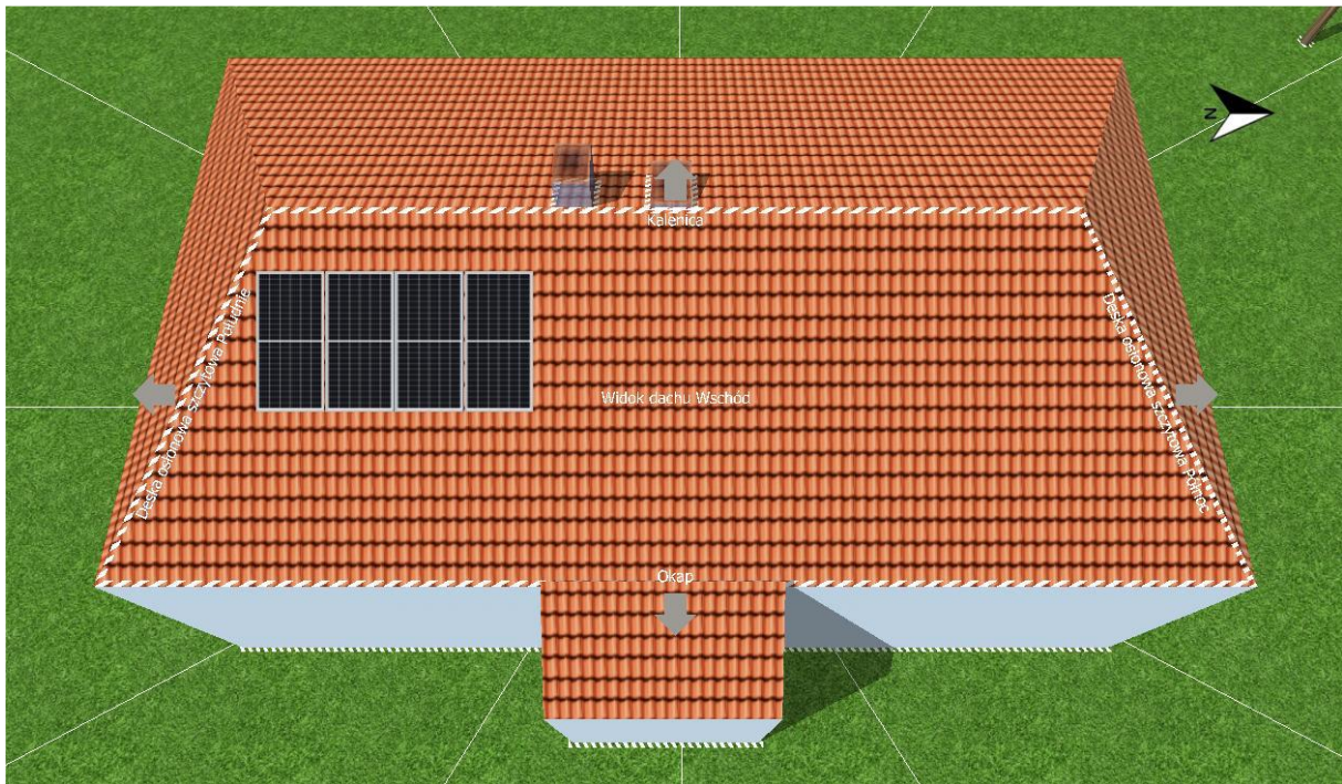
Rysunek 2. Wizualizacja instalacji fotowoltaicznej na połaciach dachowych.
